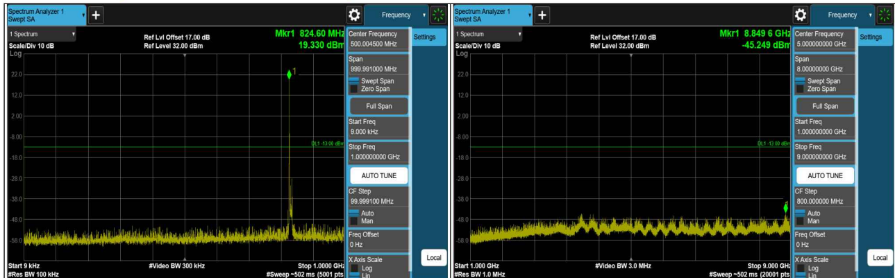
CH 26840 (829MHz)
