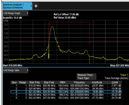
1RB#0 (822.5MHz)
