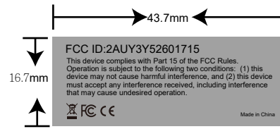
WM-2400 FCC 反銀龍貼紙 尺寸16.7x43.7mm
