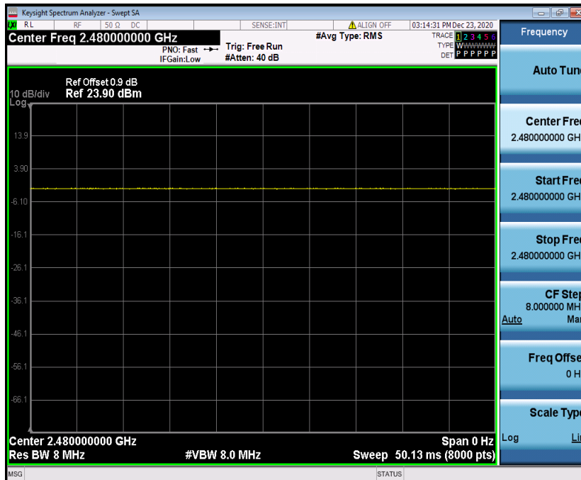
BLE_Ant1_2480
