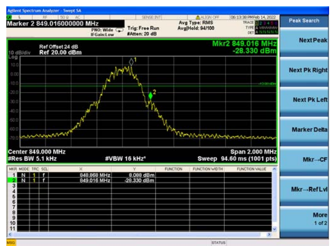
GSM850(EDGE), CH251, 848.8MHz
