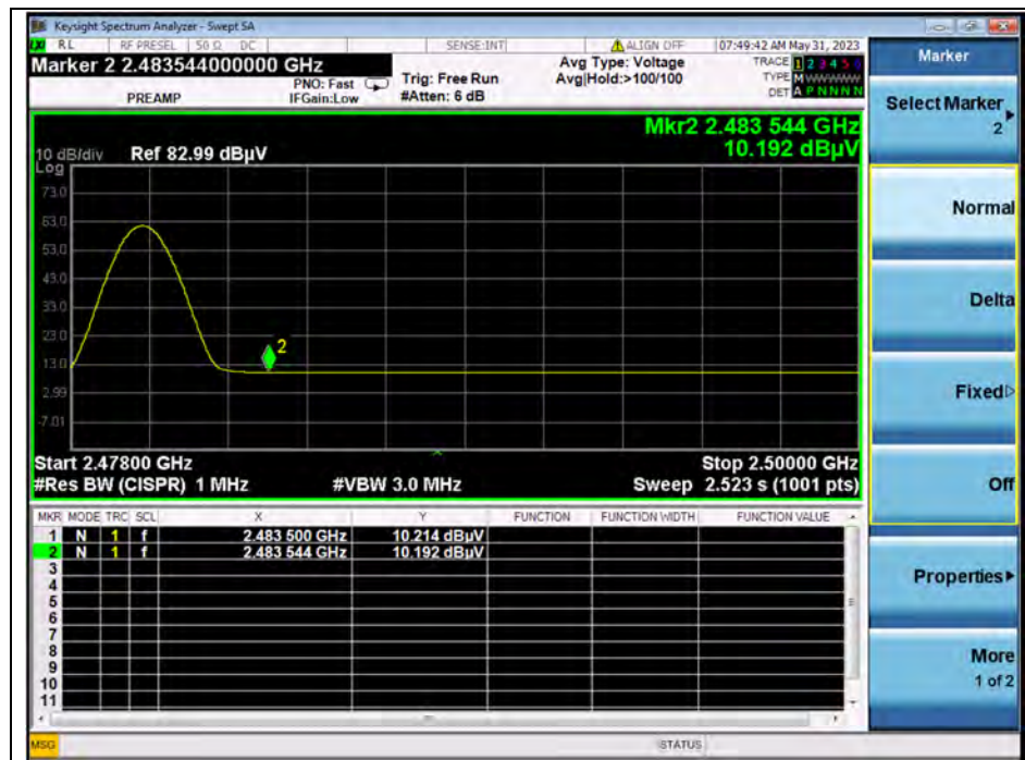
(AVERAGE, Channel 39)
