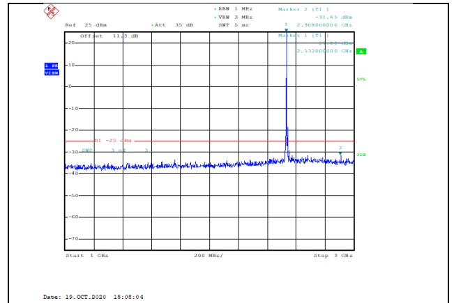
Band7-10MHz-QPSK-21100-1RB#0-Range2:1000~3000MHz--31.65-PASS
