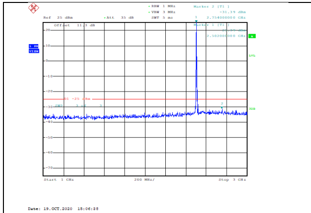
Band7-10MHz-QPSK-20800-1RB#0-Range2:1000~3000MHz--31.39-PASS
