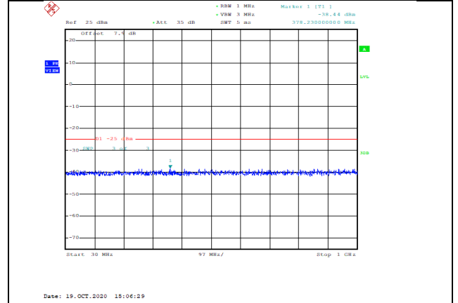
Band7-10MHz-QPSK-20800-1RB#0-Range1:30~1000MHz--38.44-PASS
