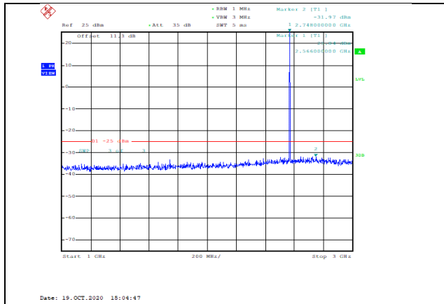
Band7-5MHz-QPSK-21425-1RB#0-Range2:1000~3000MHz--31.97-PASS
