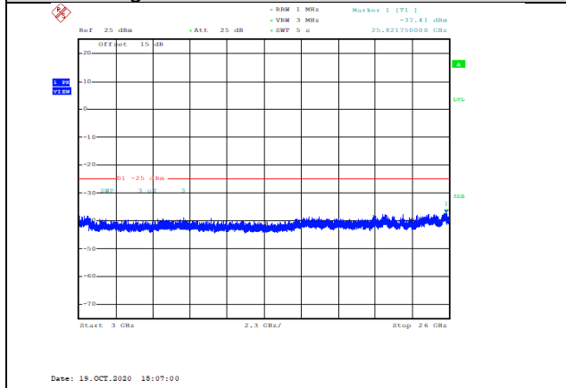
Band7-10MHz-QPSK-20800-1RB#0-Range3:3000~26000MHz--37.41-PASS
