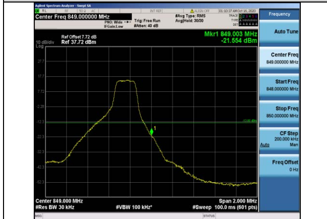
Band5-3MHz-QPSK-20635-1RB#14
