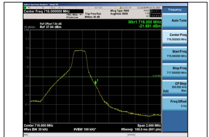
Band12-3MHz-QPSK-23165-1RB#14
