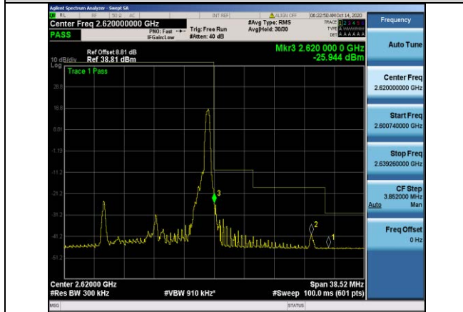
Band38-15MHz-QPSK-38175-1RB#74
