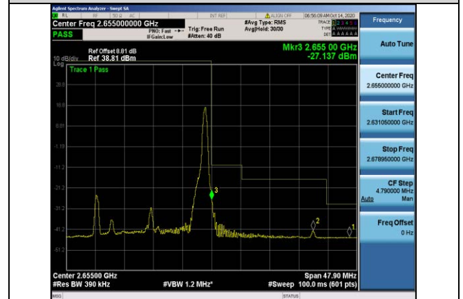
Band41-20MHz-QPSK-41140-1RB#99
