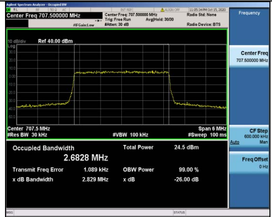
Band12-3MHz-QPSK-23095-15RB#0-2.6828
