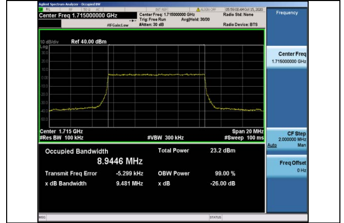
Band66-10MHz-QPSK-132022-50RB#0-8.9446
