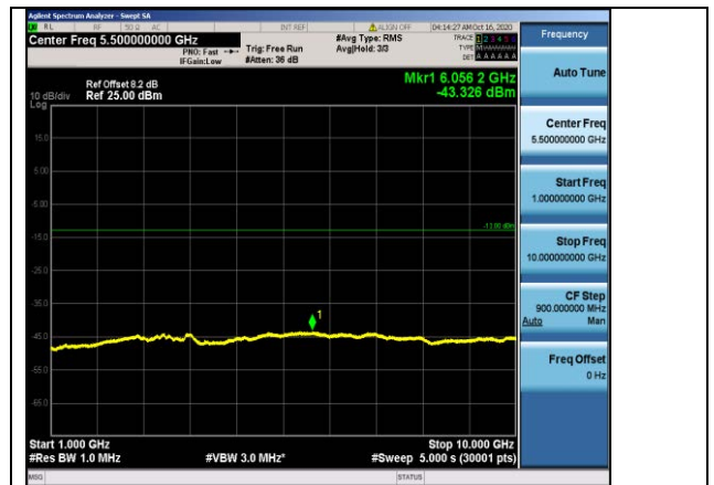
Band5-5MHz-QPSK-20525-1RB#0- Range2:1000~10000MHz
