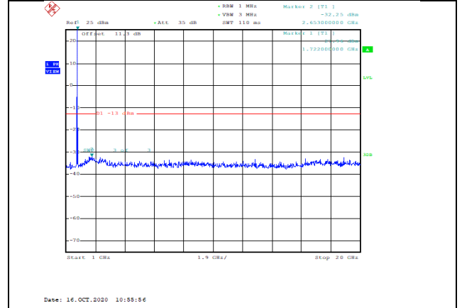
Band4-20MHz-QPSK-20175-1RB#0-Range2:1000~20000MHz--32.25-PASS
