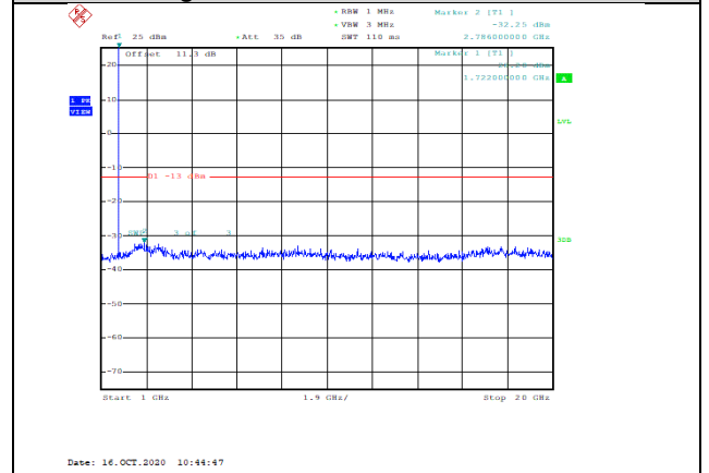
Band4-1.4MHz-QPSK-20175-1RB#0-Range2:1000~20000MHz--32.25-PASS
