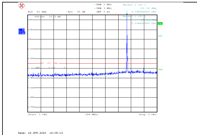
Band7-5MHz-QPSK-21100-1RB#0-Range2:1000~3000MHz--31.7-PASS
