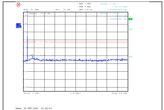
Band4-3MHz-QPSK-19965-1RB#0-Range2:1000~20000MHz--32.32-PASS
