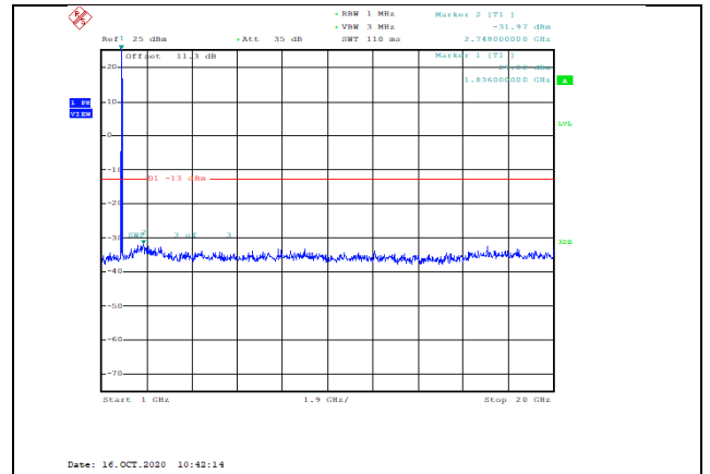
Band2-20MHz-QPSK-18700-1RB#0-Range2:1000~20000MHz--31.97-PASS
