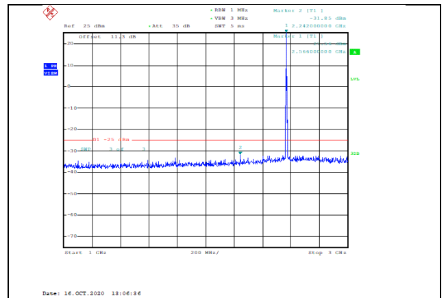
Band7-5MHz-QPSK-21425-1RB#0-Range2:1000~3000MHz--31.85-PASS
