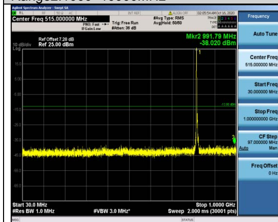
Band26-5MHz-QPSK-26765-1RB#0- Range1:30~1000MHz
