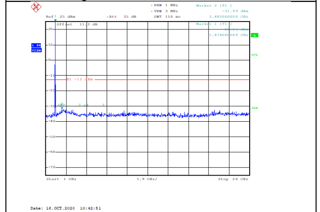
Band2-20MHz-QPSK-18900-1RB#0-Range2:1000~20000MHz--31.99-PASS
