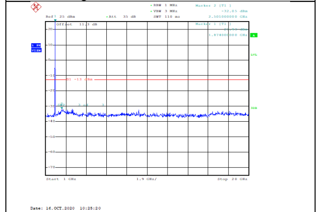
Band2-5MHz-QPSK-18900-1RB#0-Range2:1000~20000MHz--32.05-PASS
