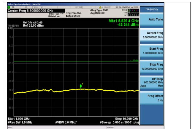
Band26-3MHz-QPSK-26775-1RB#0- Range2:1000~10000MHz
