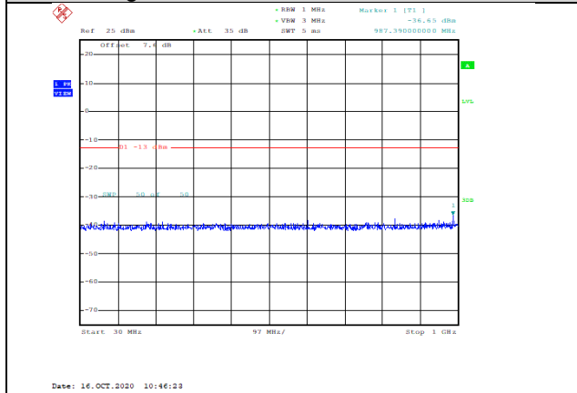
Band4-3MHz-QPSK-19965-1RB#0-Range1:30~1000MHz--36.65-PASS
