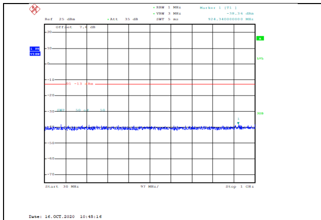
Band4-1.4MHz-QPSK-20393-1RB#0-Range1:30~1000MHz--38.36-PASS
