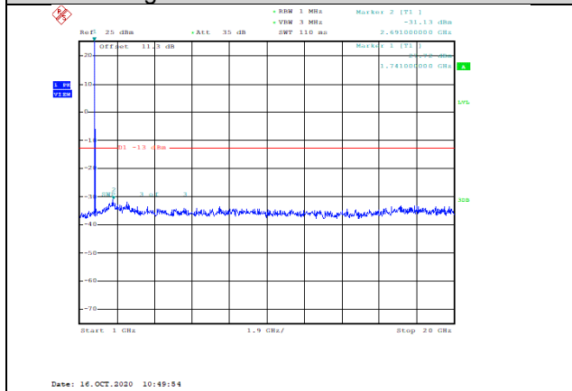
Band4-5MHz-QPSK-20375-1RB#0-Range2:1000~20000MHz--31.13-PASS
