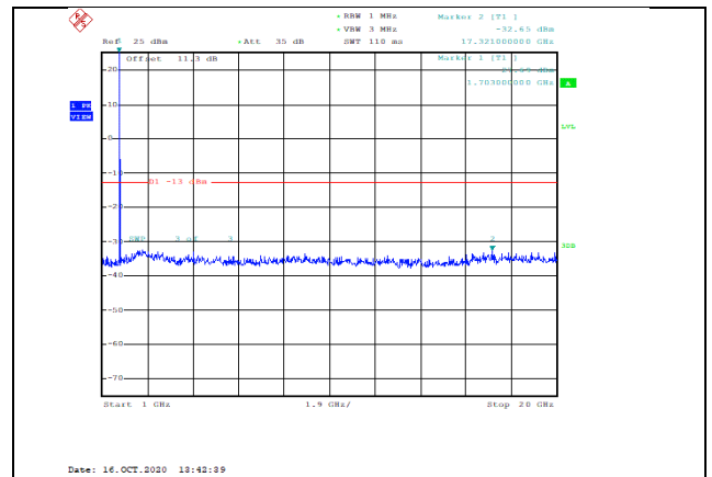
Band66-3MHz-QPSK-131987-1RB#0-Range2:1000~20000MHz--32.65-PASS
