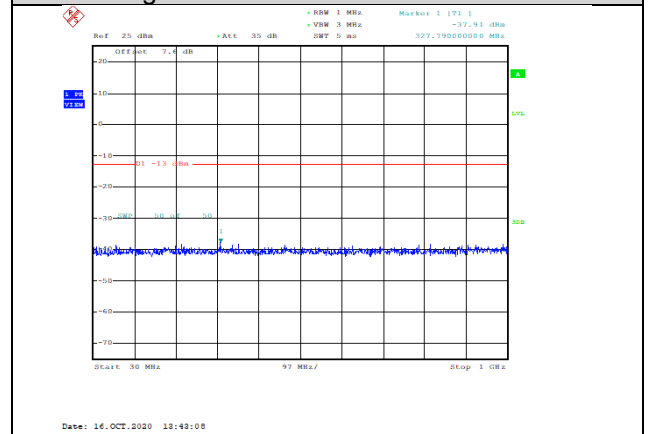
Band66-3MHz-QPSK-132322-1RB#0-Range1:30~1000MHz--37.91-PASS
