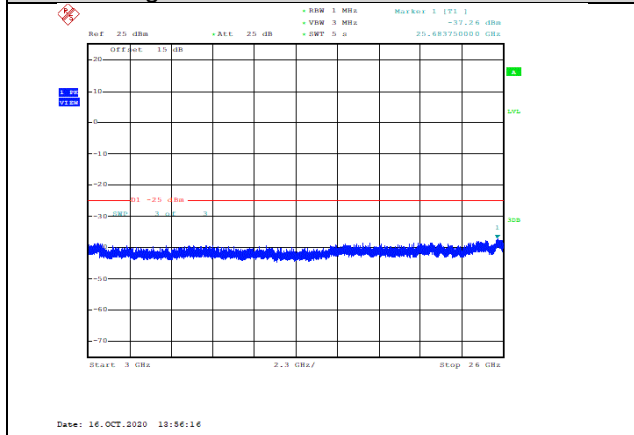
Band41-5MHz-QPSK-40590-1RB#0-Range3:3000~26000MHz--37.26-PASS
