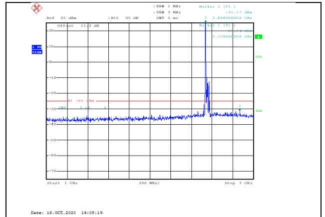
Band41-20MHz-QPSK-40140-1RB#0-Range2:1000~3000MHz--31.57-PASS
