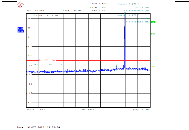
Band41-5MHz-QPSK-40590-1RB#0-Range2:1000~3000MHz--31.89-PASS
