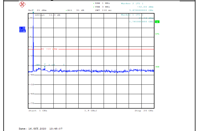
Band66-10MHz-QPSK-132322-1RB#0-Range2:1000~20000MHz--32-PASS
