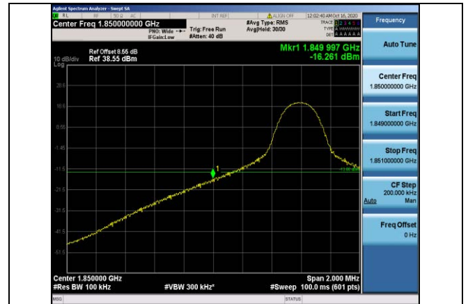
Band2-10MHz-QPSK-18650-1RB#0
