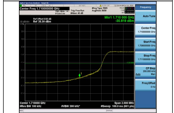
Band4-10MHz-QPSK-20000-50RB#0
