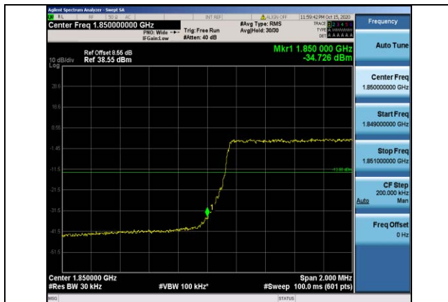
Band2-3MHz-QPSK-18615-15RB#0
