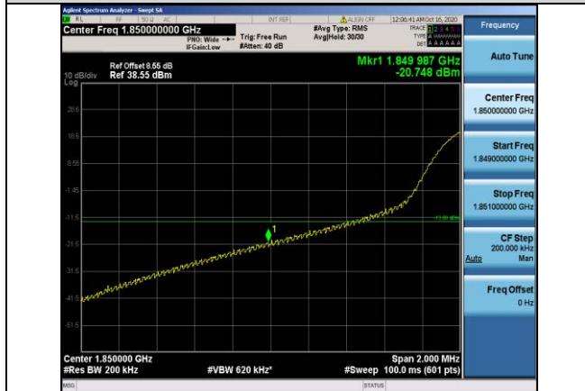
Band2-20MHz-QPSK-18700-1RB#0
