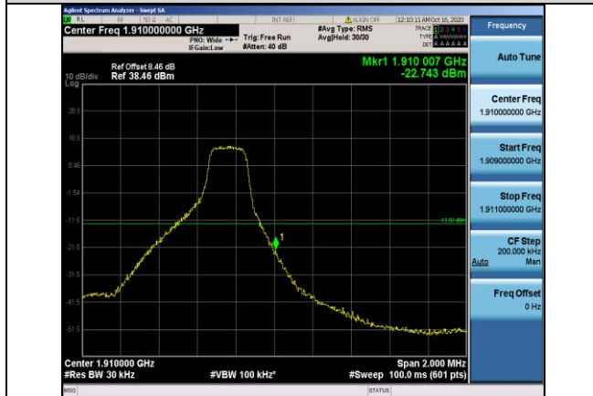
Band2-3MHz-QPSK-19185-1RB#14
