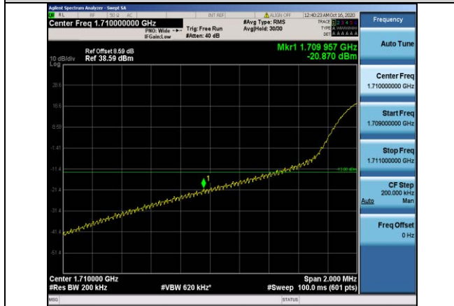
Band4-20MHz-QPSK-20050-1RB#0
