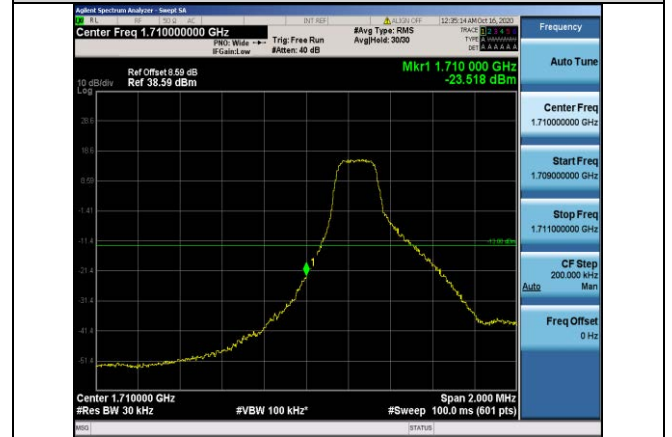
Band4-3MHz-QPSK-19965-1RB#0
