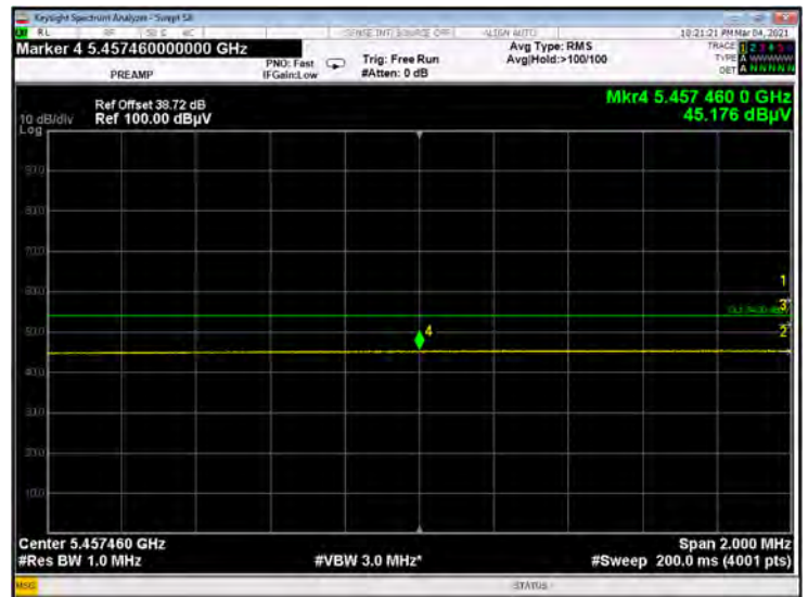
U-NII-2C 11ac80 CH106 AV
