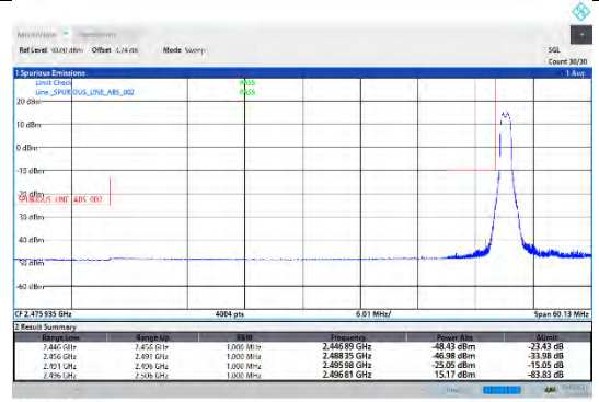
CA_41C-20MHz-20MHz-QPSK-QPSK-39750-39948-1RB#0-0RB#0
