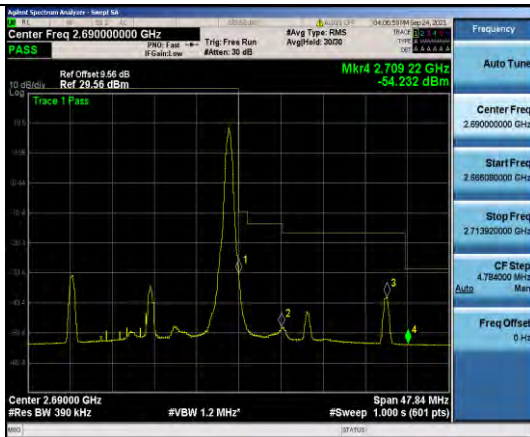
Band41-20MHz-16QAM-41490-1RB#99
