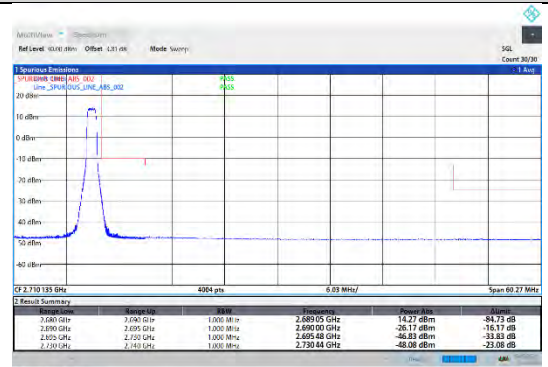
CA_41C-20MHz-20MHz-16QAM-16QAM-41292-41490-0RB#0-1RB#99
