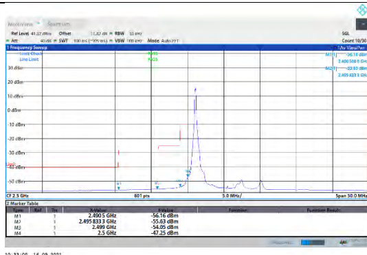
CA_7C-10MHz-20MHz-QPSK-QPSK-20805-20949-1RB#0-0RB#0
