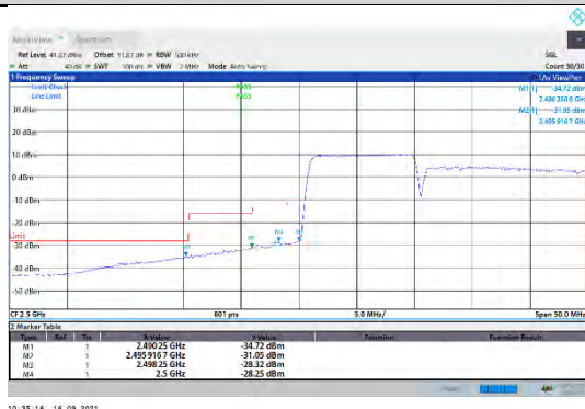
CA_7C-10MHz-20MHz-QPSK-QPSK-20805-20949-50RB#0-100RB#0
