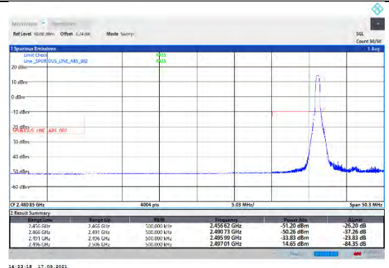
CA_41C-20MHz-10MHz-QPSK-QPSK-39750-39894-1RB#0-0RB#0
