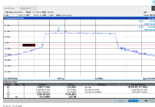
N41-30kHz-20MHz-CP-QPSK-Mid-Outer_Full---PASS
