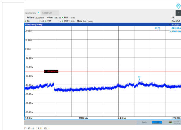
Band41-15MHz-QPSK-41165-1RB#0- Range3:3000~27000MHz
