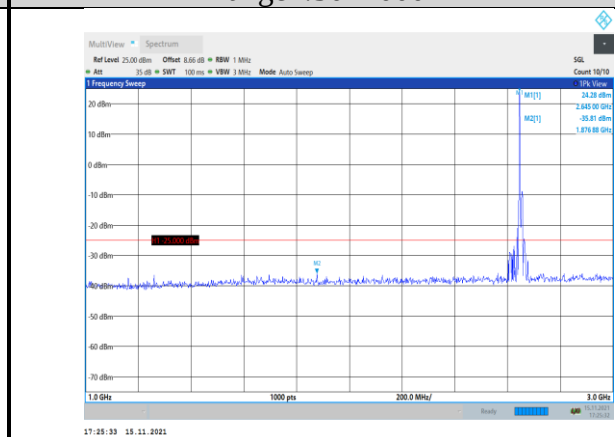
Band41-10MHz-QPSK-41190-1RB#0- Range2:1000~3000MHz
