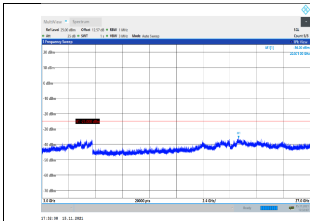
Band41-20MHz-QPSK-40140-1RB#0- Range3:3000~27000MHz
