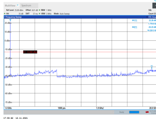
Band66-5MHz-QPSK-132647-1RB#0- Range2:1000~20000MHz
