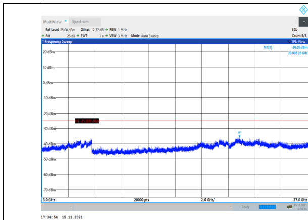
Band41-20MHz-QPSK-41140-1RB#0- Range3:3000~27000MHz
