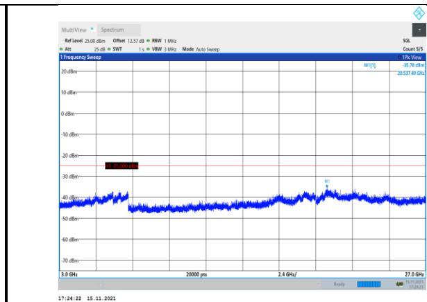
Band41-10MHz-QPSK-40590-1RB#0- Range3:3000~27000MHz
