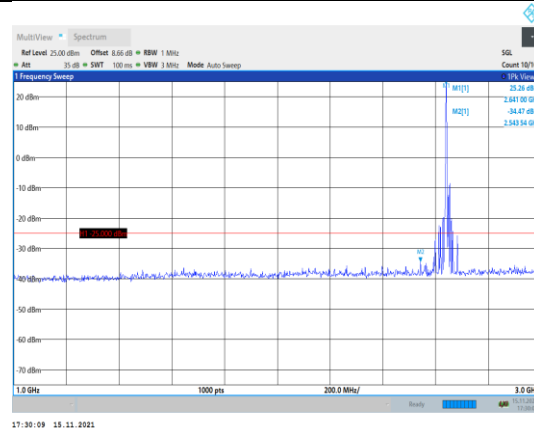
Band41-15MHz-QPSK-41165-1RB#0- Range2:1000~3000MHz
