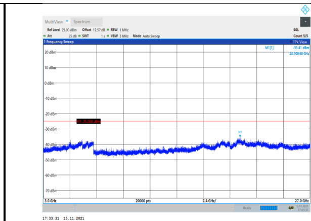
Band41-20MHz-QPSK-40590-1RB#0- Range3:3000~27000MHz
