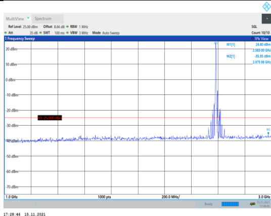
Band41-15MHz-QPSK-40590-1RB#0- Range2:1000~3000MHz
