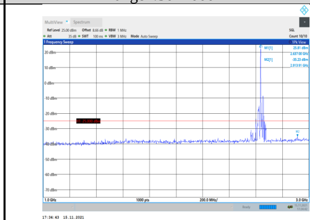
Band41-20MHz-QPSK-41140-1RB#0- Range2:1000~3000MHz
