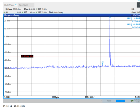
Band41-5MHz-QPSK-40065-1RB#0- Range2:1000~3000MHz
