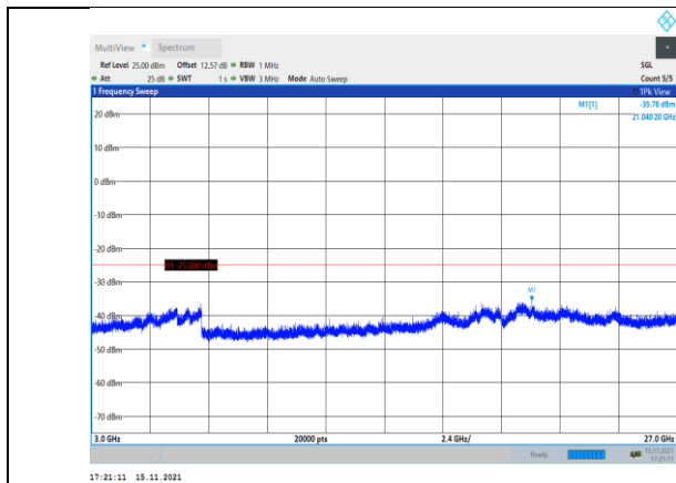
Band41-5MHz-QPSK-41215-1RB#0- Range3:3000~27000MHz
