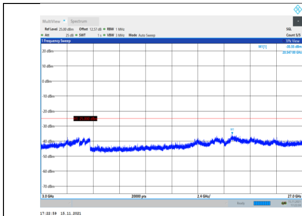
Band41-10MHz-QPSK-40090-1RB#0- Range3:3000~27000MHz
