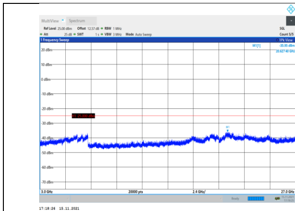
Band41-5MHz-QPSK-40065-1RB#0- Range3:3000~27000MHz
