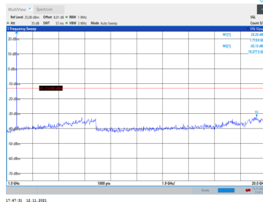
Band66-3MHz-QPSK-131987-1RB#0- Range2:1000~20000MHz
