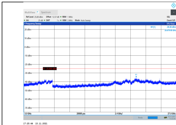
Band41-10MHz-QPSK-41190-1RB#0- Range3:3000~27000MHz
