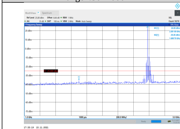
Band41-20MHz-QPSK-40590-1RB#0- Range2:1000~3000MHz
