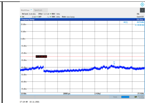
Band41-5MHz-QPSK-40590-1RB#0- Range3:3000~27000MHz
