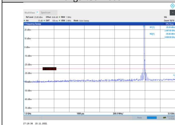
Band41-5MHz-QPSK-40590-1RB#0- Range2:1000~3000MHz
