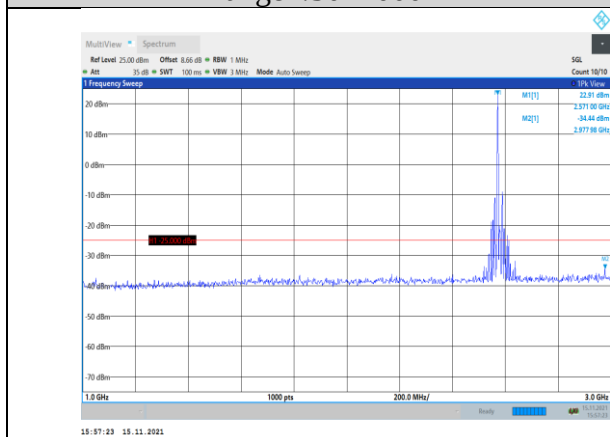
Band38-20MHz-16QAM-37850-1RB#0- Range2:1000~3000MHz
