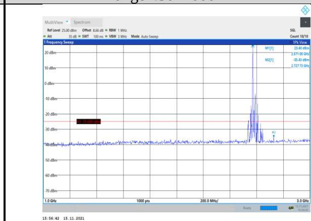
Band38-20MHz-QPSK-37850-1RB#0- Range2:1000~3000MHz
