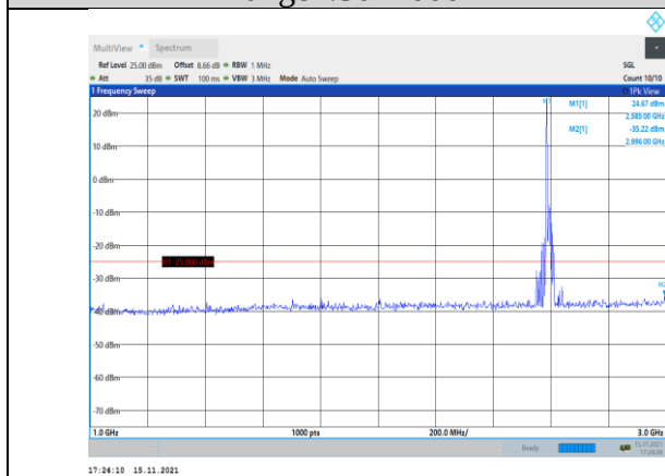
Band41-10MHz-QPSK-40590-1RB#0- Range2:1000~3000MHz
