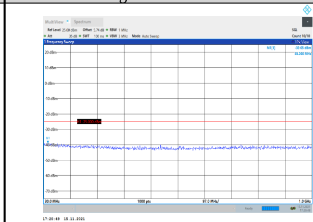
Band41-5MHz-QPSK-41215-1RB#0- Range1:30~1000MHz
