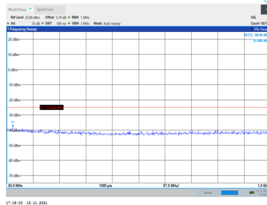
Band41-5MHz-QPSK-40065-1RB#0- Range1:30~1000MHz
