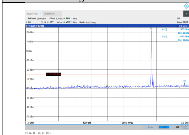
Band41-5MHz-16QAM-40065-1RB#0- Range2:1000~3000MHz
