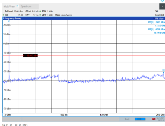
Band66-20MHz-QPSK-132322-1RB#0- Range2:1000~20000MHz
