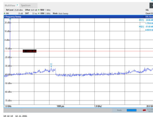
Band66-20MHz-QPSK-132572-1RB#0- Range2:1000~20000MHz
