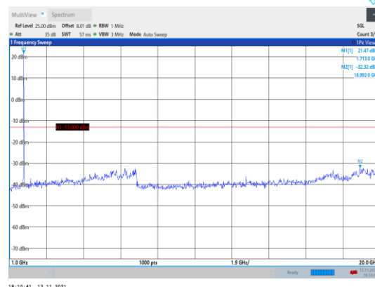
Band66-20MHz-16QAM-132072-1RB#0- Range2:1000~20000MHz
