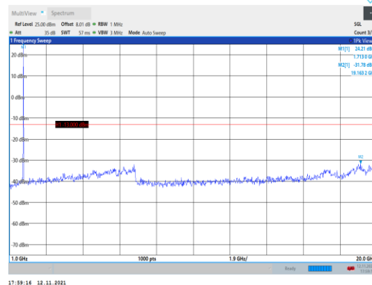
Band66-10MHz-QPSK-132022-1RB#0- Range2:1000~20000MHz
