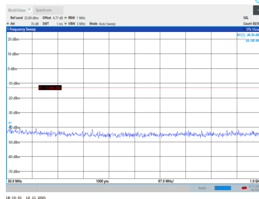
Band66-20MHz-QPSK-132072-1RB#0- Range1:30~1000MHz
