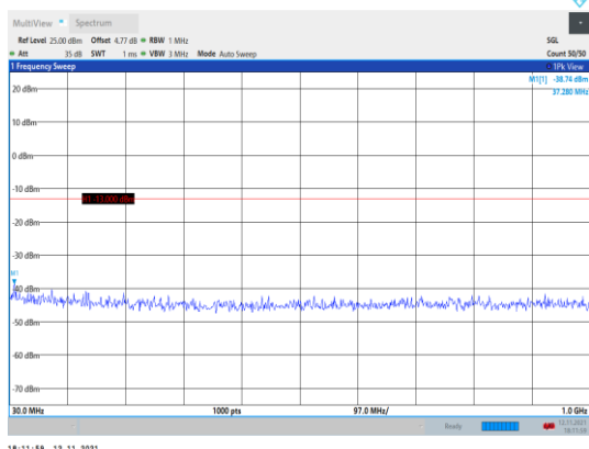
Band66-20MHz-QPSK-132572-1RB#0- Range1:30~1000MHz
