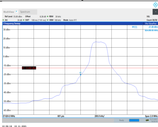
Band5-3MHz-QPSK-20415-1RB#0
