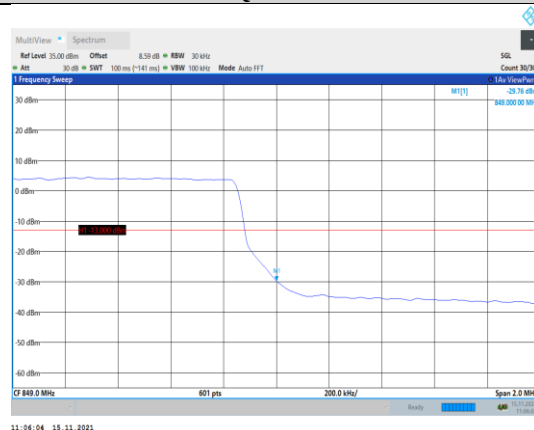
Band5-3MHz-QPSK-20635-15RB#0
