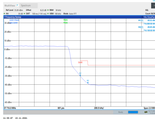
Band12-3MHz-QPSK-23165-15RB#0
