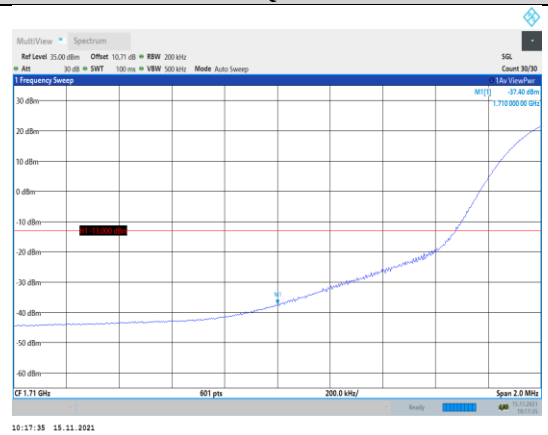
Band4-20MHz-QPSK-20050-1RB#0
