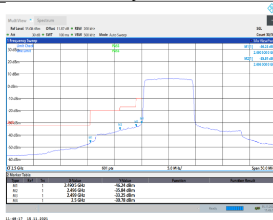
Band7-10MHz-QPSK-20800-50RB#0
