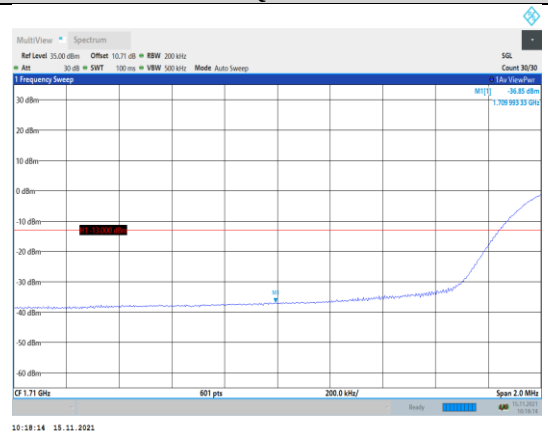
Band4-20MHz-QPSK-20050-100RB#0
