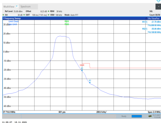
Band12-3MHz-QPSK-23165-1RB#14
