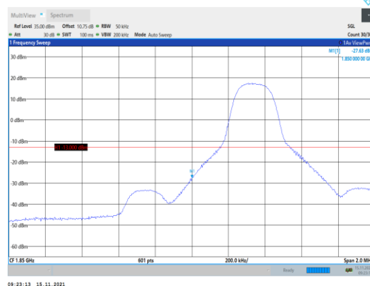
Band2-5MHz-QPSK-18625-1RB#0
