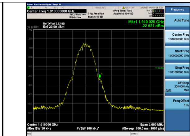
GPRS1900-810-0
