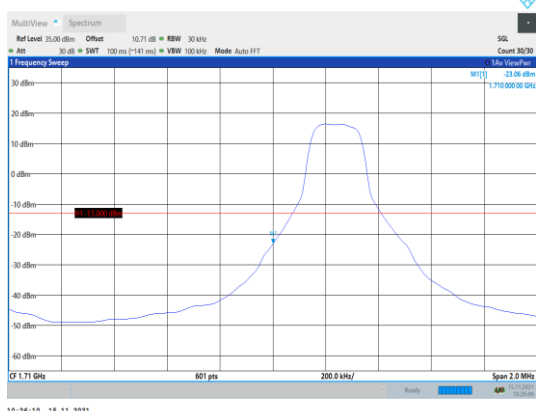
Band4-3MHz-QPSK-19965-1RB#0
