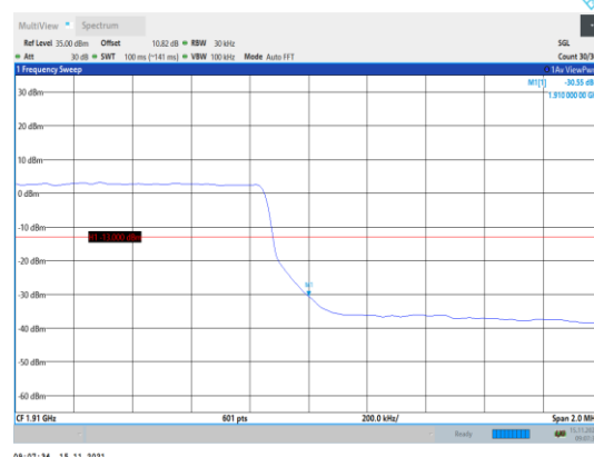
Band2-3MHz-QPSK-19185-15RB#0
