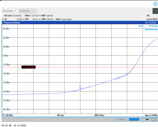
Band2-20MHz-16QAM-18700-1RB#0
