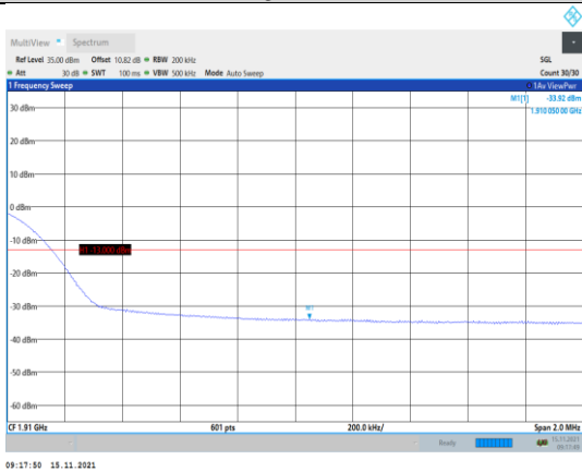
Band2-20MHz-QPSK-19100-100RB#0
