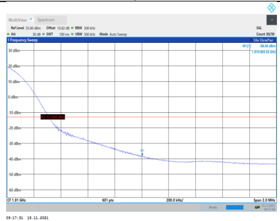
Band2-20MHz-16QAM-19100-1RB#99
