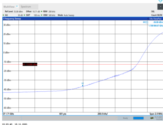
Band66-20MHz-QPSK-132072-1RB#0
