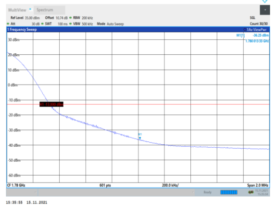
Band66-20MHz-QPSK-132572-1RB#99
