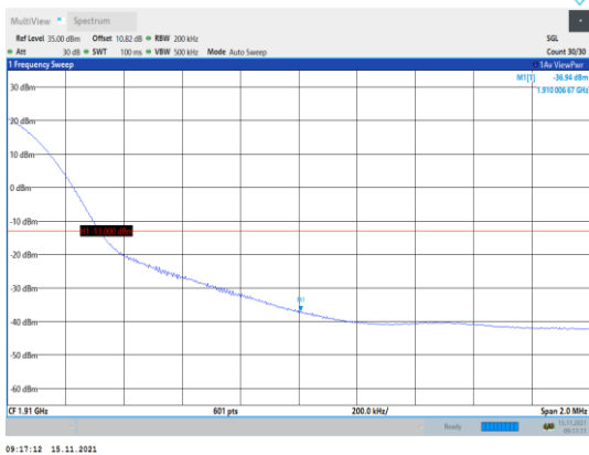
Band2-20MHz-QPSK-19100-1RB#99
