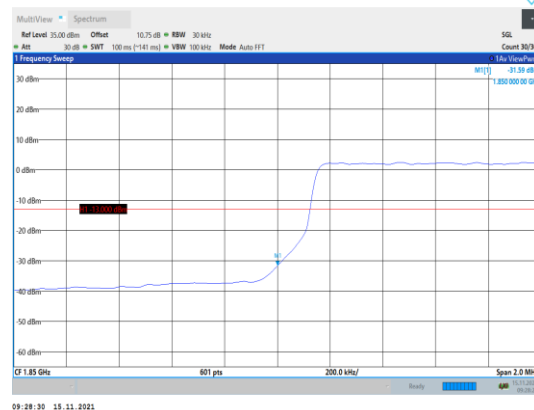
Band2-3MHz-QPSK-18615-15RB#0
