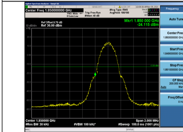
GPRS1900-512-0
