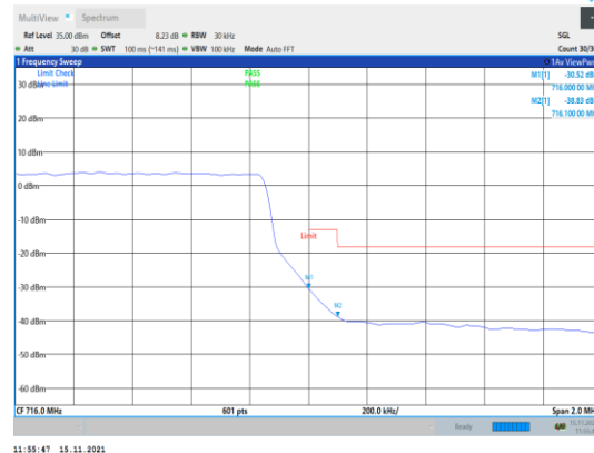
Band12-3MHz-QPSK-23165-15RB#0
