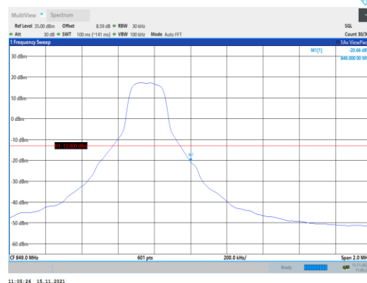
Band5-3MHz-QPSK-20635-1RB#14
