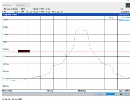
Band5-3MHz-QPSK-20415-1RB#0
