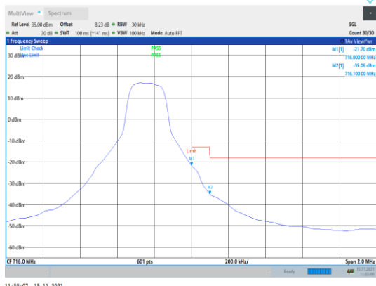
Band12-3MHz-QPSK-23165-1RB#14
