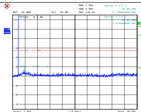
Band2-3MHz-QPSK-18900-1RB#0-Range2:1000~20000MHz
