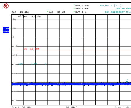
GSM1900-512-0-30~1000MHz
