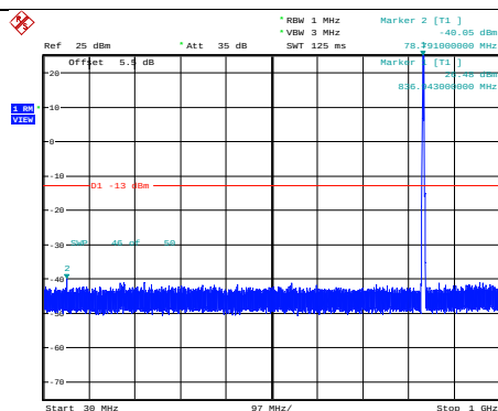
EGPRS850-128-8-30~1000MHz
