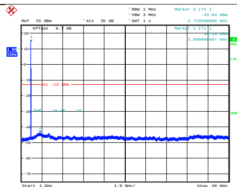
GSM1900-661-0-1000~20000MHz
