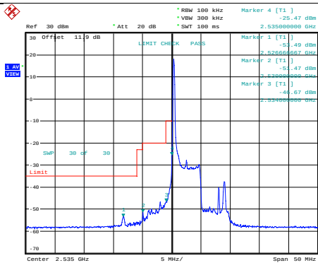
Band41-5MHz-QPSK-40065-1RB#0
