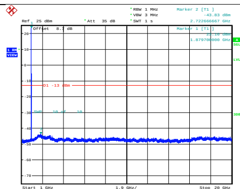
EGPRS1900-661-2-1000~20000MHz
