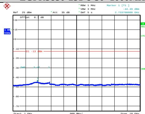
EGPRS850-251-8-1000~10000MHz
