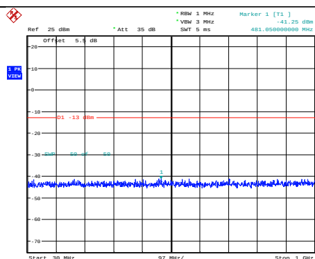
Band4-3MHz-QPSK-19965-1RB#0- Range1:30~1000MHz
