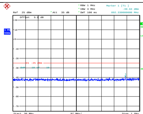
Band7-10MHz-QPSK-20800-1RB#0- Range1:30~1000MHz
