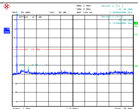
Band4-5MHz-QPSK-20175-1RB#0- Range2:1000~20000MHz
