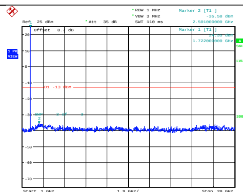
Band4-3MHz-QPSK-20175-1RB#0- Range2:1000~20000MHz
