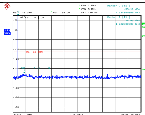
Band4-1.4MHz-QPSK-20175-1RB#0- Range2:1000~20000MHz
