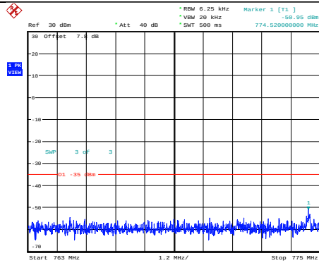
Band13-5MHz-QPSK-23230-1RB#0-Range3:763~775MHz
