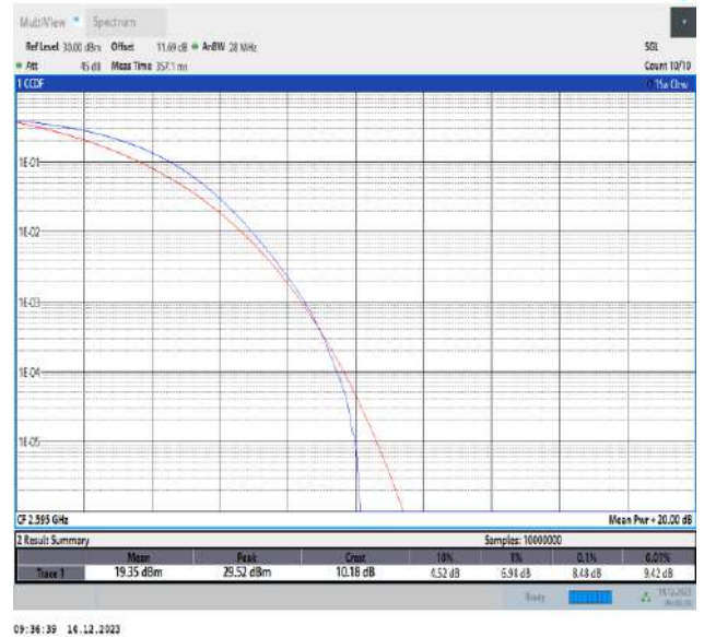
38-38-20MHz-20MHz-QPSK-QPSK-37901-38099-100RB#0-100RB#0-PASS
