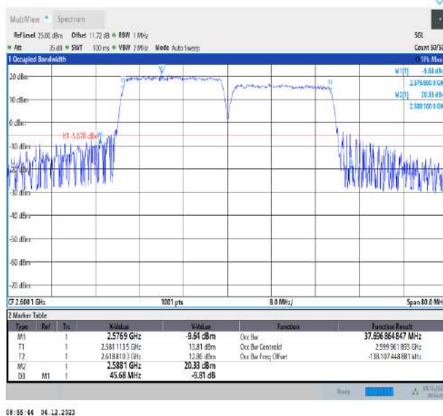
38-38-20MHz-20MHz-QPSK-QPSK-37952-38150-100RB#0-100RB#0-PASS
