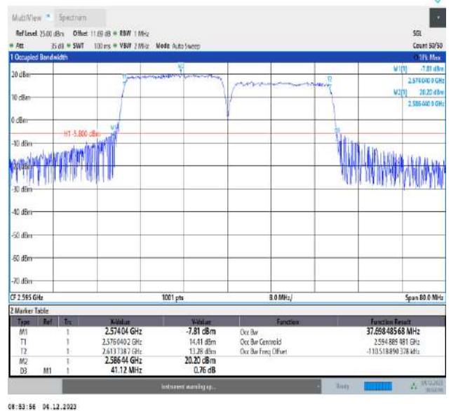
38-38-20MHz-20MHz-QPSK-QPSK-37901-38099-100RB#0-100RB#0-PASS
