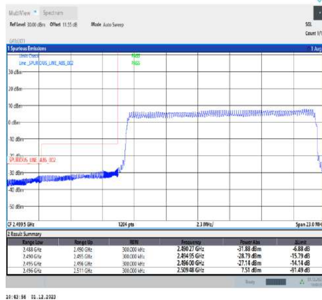
Band41_15MHz_QPSK_39725_75RB#0
