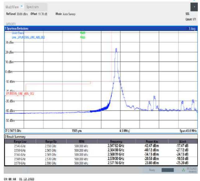
Band38_20MHz_QPSK_37850_1RB#0
