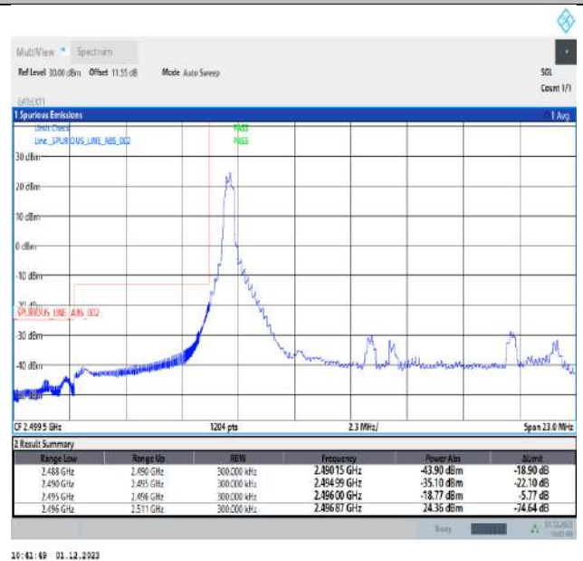
Band41_15MHz_QPSK_39725_1RB#0
