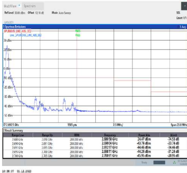
Band41_10MHz_QPSK_41540_1RB#0
