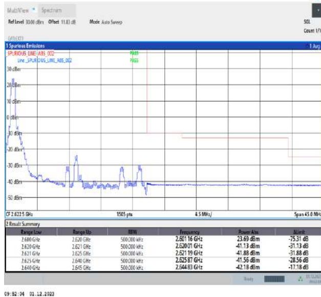
Band38_20MHz_QPSK_38150_1RB#0
