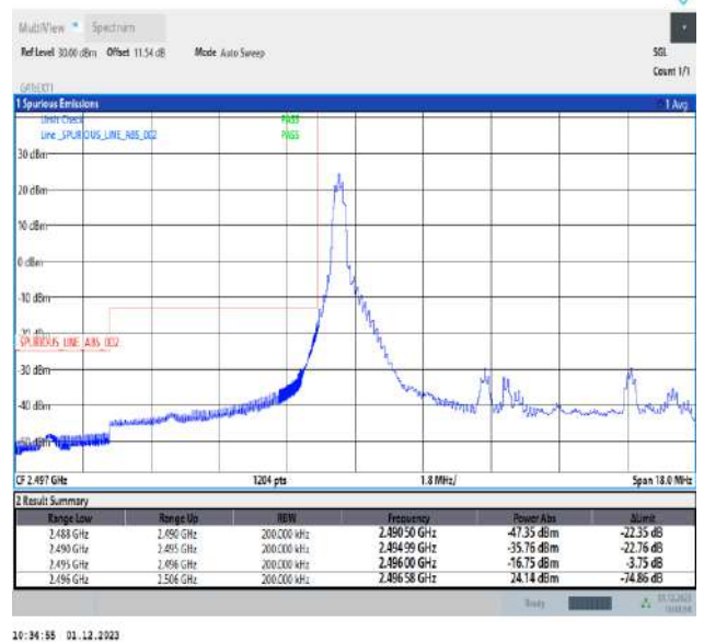
Band41_10MHz_QPSK_39700_1RB#0
