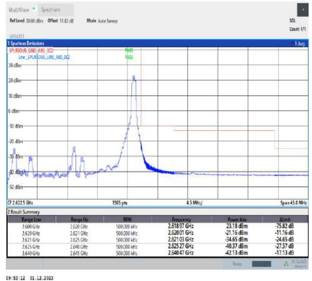
Band38_20MHz_QPSK_38150_1RB#99
