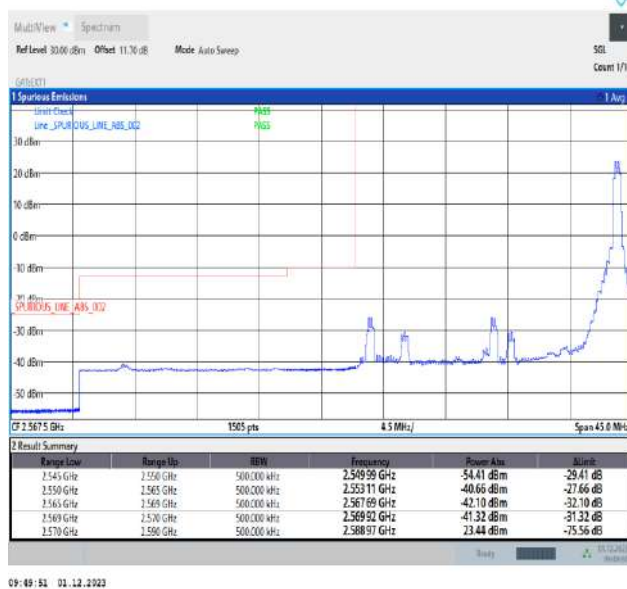
Band38_20MHz_QPSK_37850_1RB#99
