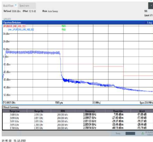
Band41_10MHz_QPSK_41540_50RB#0
