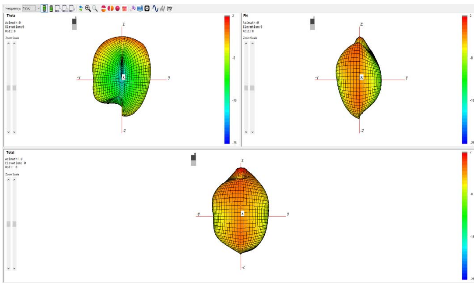
LTE ANT1 (2300~2400)
