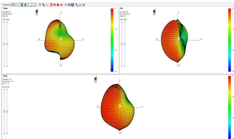
LTE ANT1 (2490~2690)
