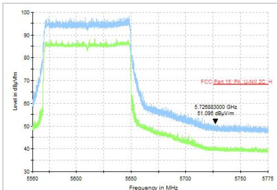
Fig. 42 Band Edges (802.11be-EHT80, CH122 5610MHz), MIMO
