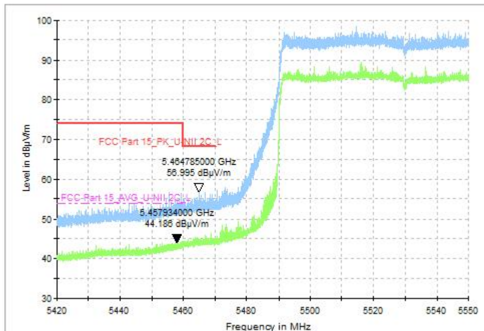
Fig. 41 Band Edges (802.11be-EHT80, CH106 5530MHz), MIMO
