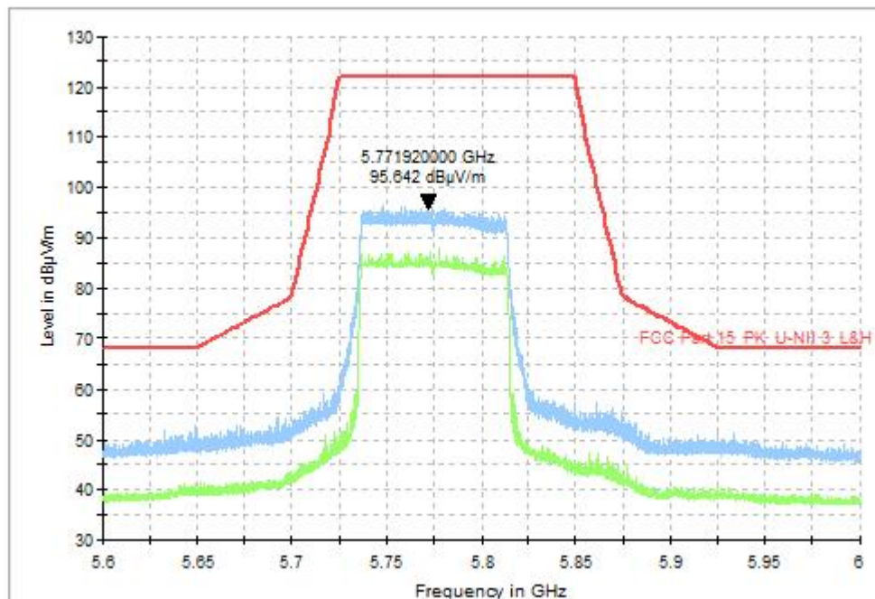
Fig. 43 Band Edges (802.11be-EHT80, CH155 5775MHz), MIMO
