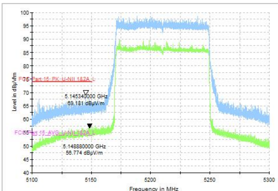
Fig. 39 Band Edges (802.11be-EHT80, CH42 5210MHz), MIMO
