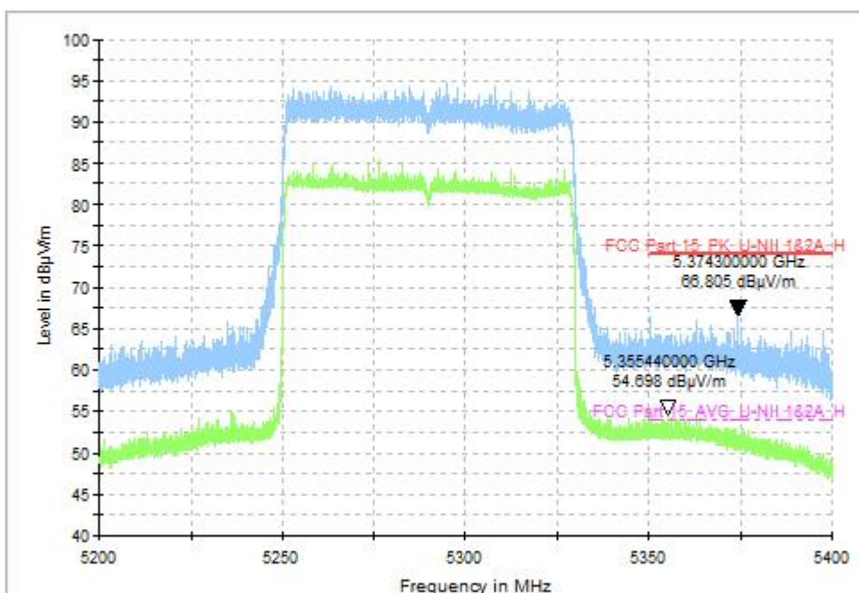
Fig. 40 Band Edges (802.11be-EHT80, CH58 5290MHz), MIMO
