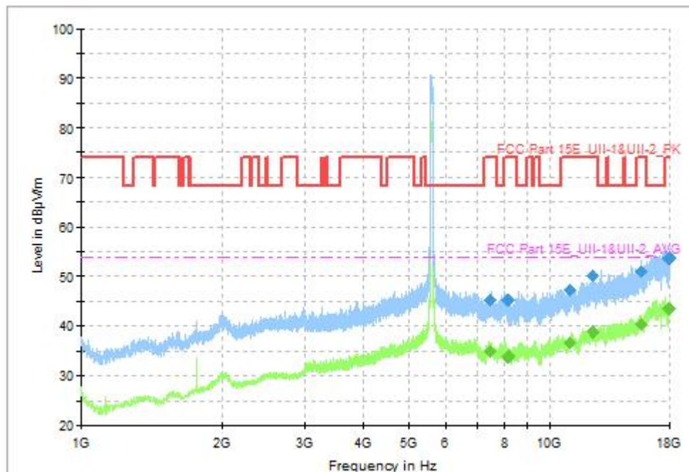
Fig. 70 Transmitter Spurious Emission (802.11be-EHT80, CH122 5610MHz, 1GHz-18GHz), MIMO
