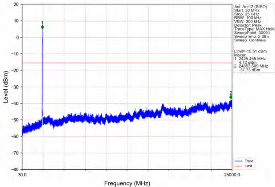
802.11n(HT40)_MCH_2437MHz_Ant12 (SISO)_NTNV
