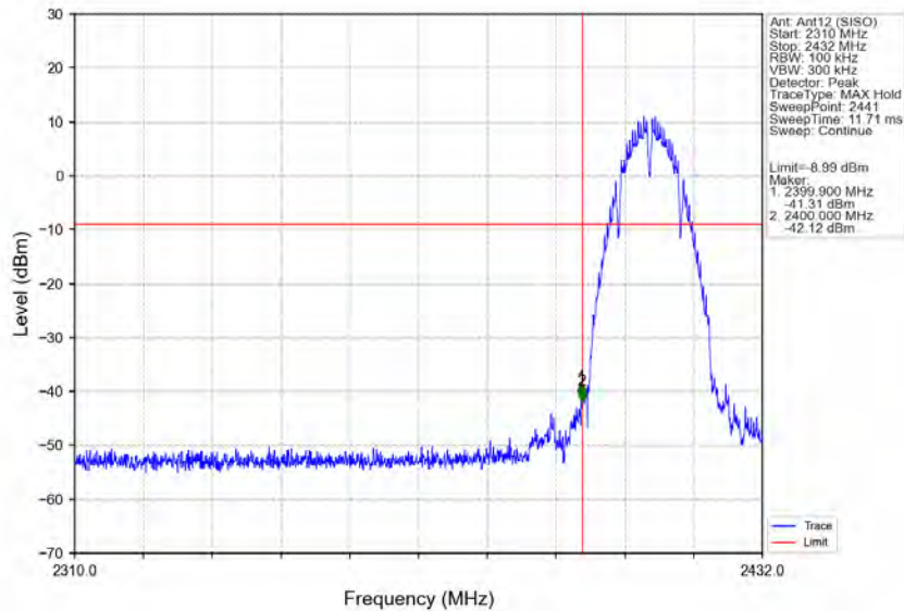
802.11b_LCH_2412MHz_Ant12 (SISO)_NTNV
