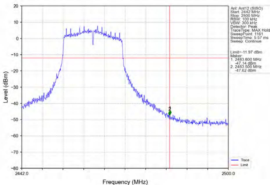
802.11g_HCH_2462MHz_Ant12 (SISO)_NTNV
