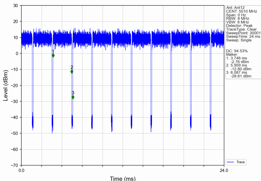
802.11ax(HEW40)_LCH_5510MHz_RU484_Left_Ant12_NTNV
