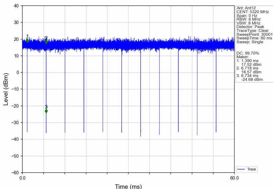
802.11n(HT20)_HCH_5320MHz_Ant12_NTNV
