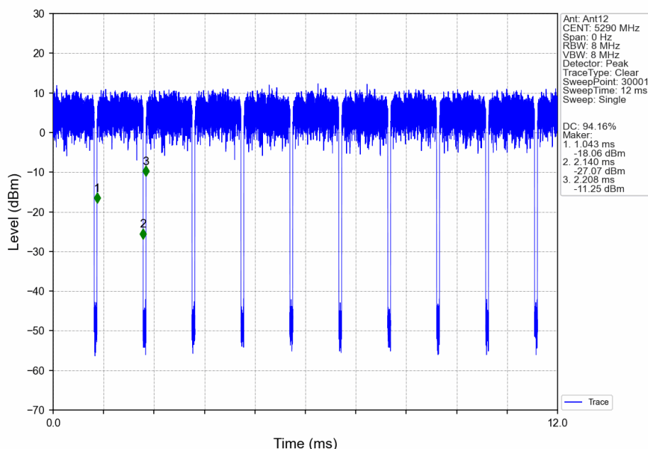
802.11ax(HEW80)_MCH_5290MHz_RU996_Left_Ant12_NTNV
