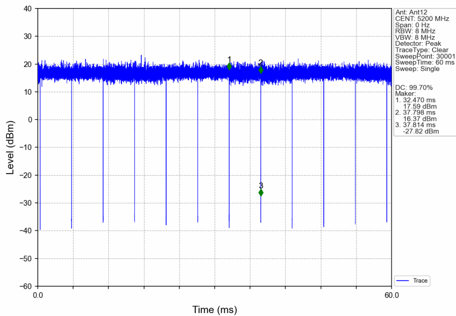
802.11n(HT20)_MCH_5200MHz_Ant12_NTNV
