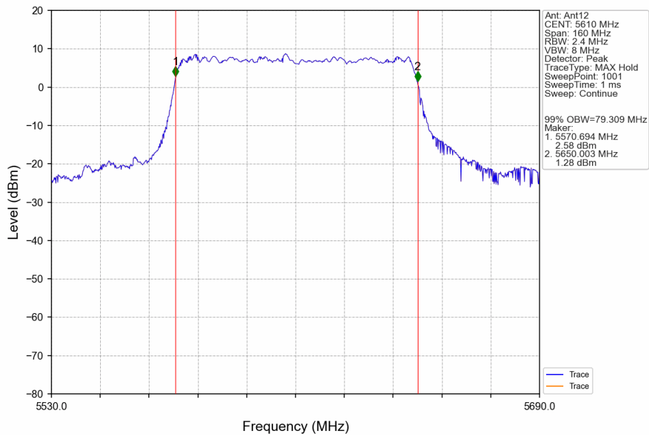
802.11ax(HEW80)_HCH_5610MHz_RU996_Left_Ant12_NTNV
