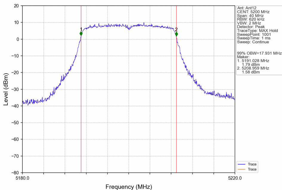
802.11n(HT20)_MCH_5200MHz_Ant12_NTNV
