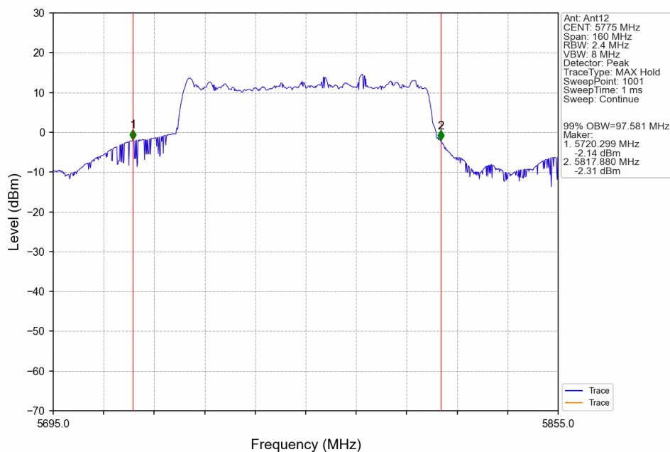
802.11ax(HEW80)_MCH_5775MHz_RU996_Left_Ant12_NTNV
