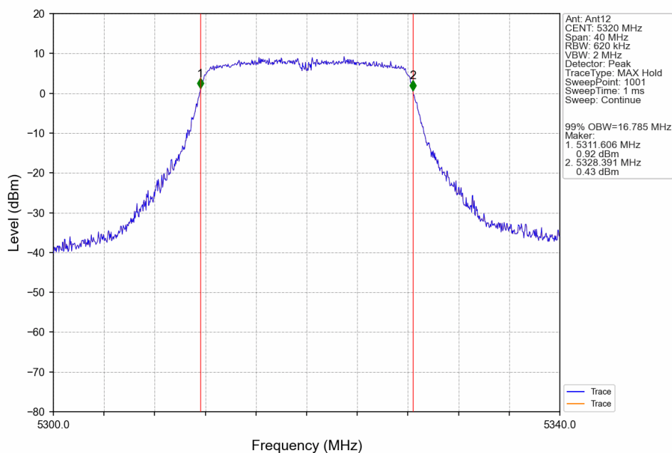
802.11a_HCH_5320MHz_Ant12_NTNV
