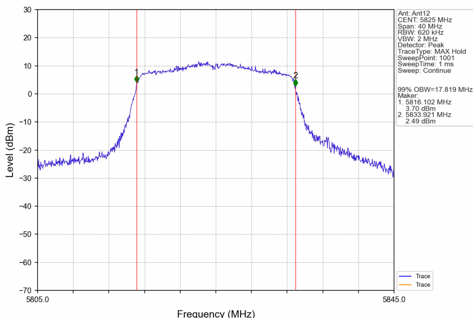
802.11n(HT20)_HCH_5825MHz_Ant12_NTNV
