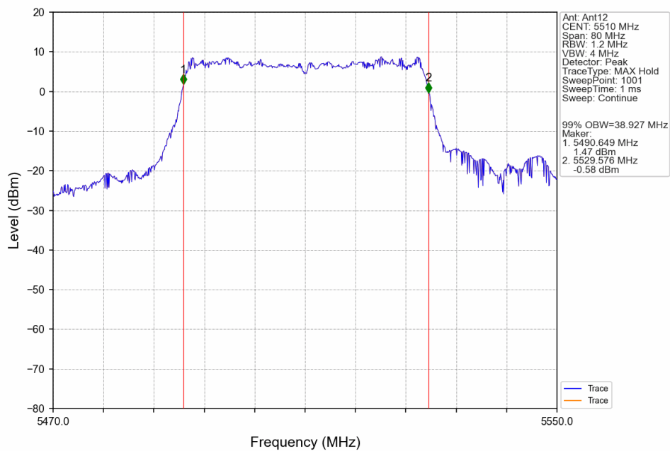
802.11ax(HEW40)_LCH_5510MHz_RU484_Left_Ant12_NTNV
