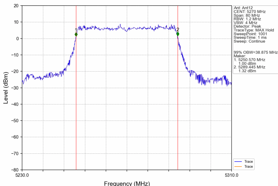
802.11ax(HEW40)_LCH_5270MHz_RU484_Left_Ant12_NTNV
