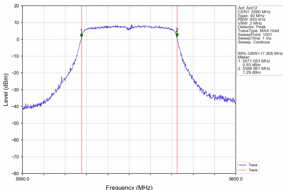
802.11n(HT20)_MCH_5580MHz_Ant12_NTNV
