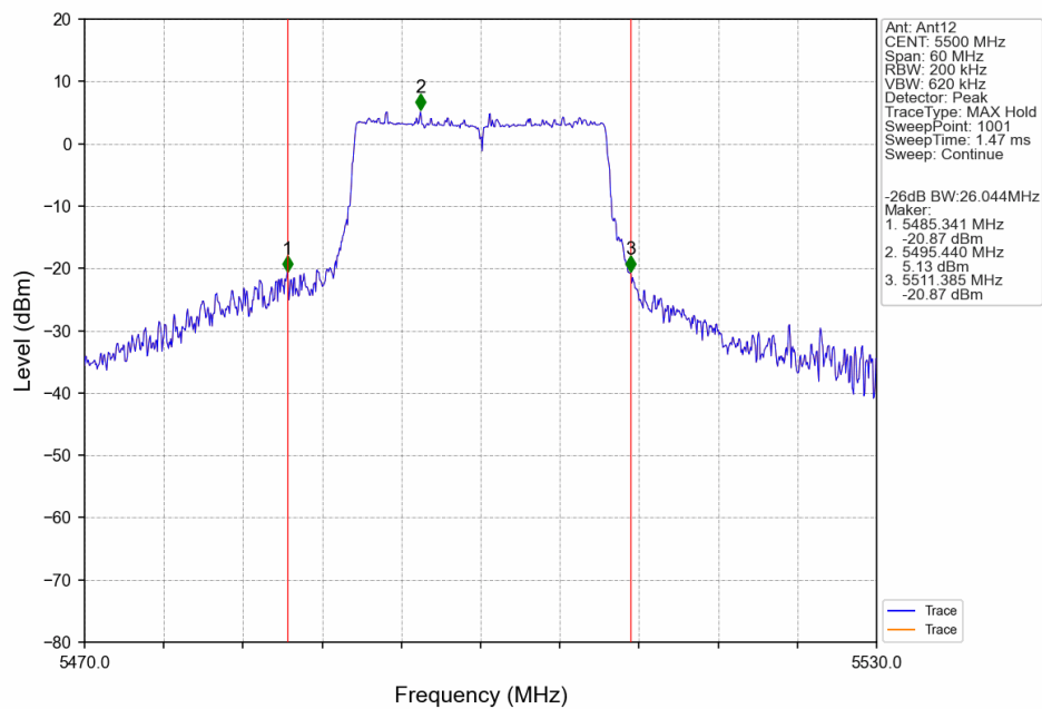
802.11ax(HEW20)_LCH_5500MHz_RU242_Left_Ant12_NTNV
