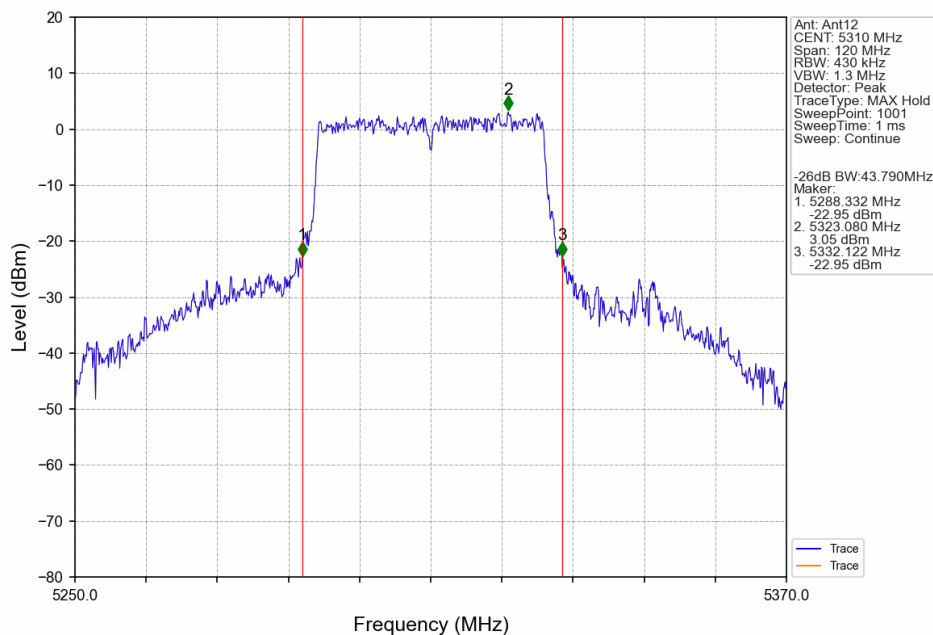
802.11ax(HEW40)_HCH_5310MHz_RU484_Left_Ant12_NTNV
