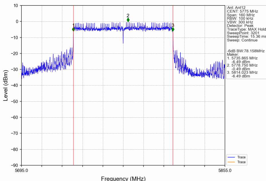
802.11ax(HEW80)_MCH_5775MHz_RU996_Left_Ant12_NTNV
