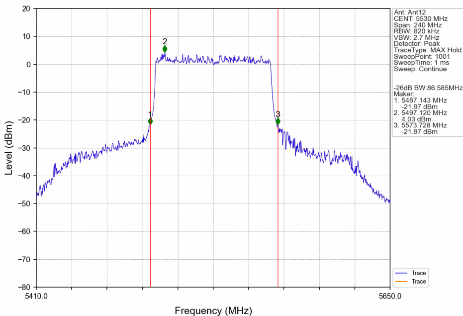
802.11ax(HEW80)_LCH_5530MHz_RU996_Left_Ant12_NTNV
