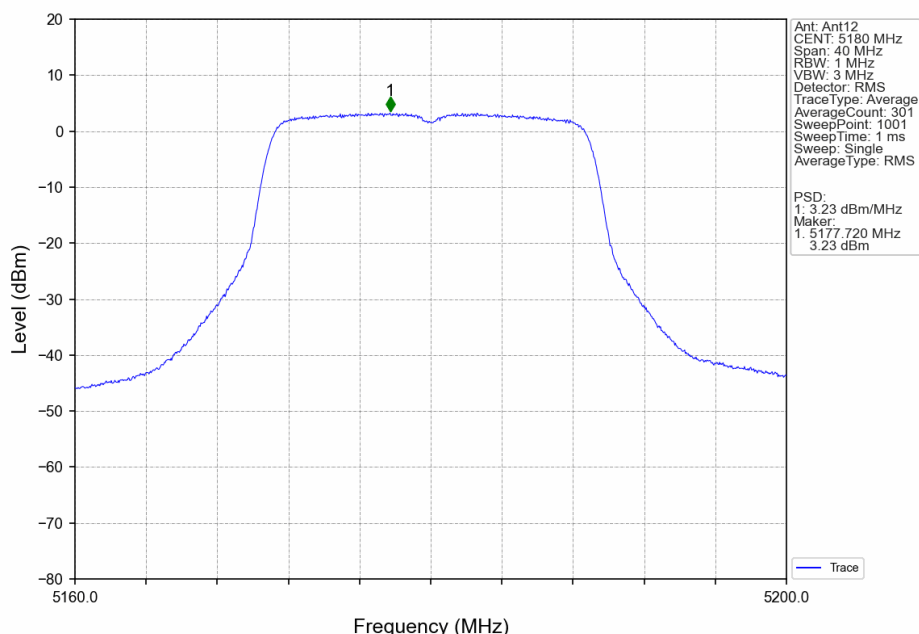
802.11ac(VHT20)_LCH_5180MHz_Ant12_NTNV
