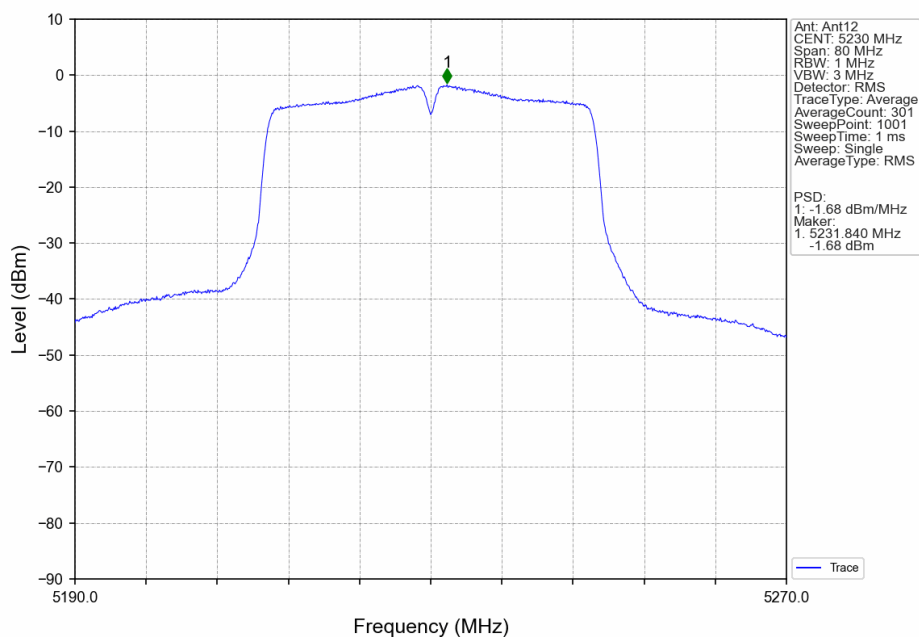
802.11ac(VHT40)_HCH_5230MHz_Ant12_NTNV
