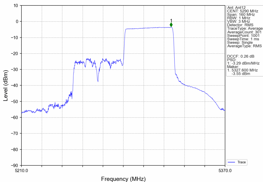
802.11ax(HEW80)_MCH_5290MHz_RU484_Right_Ant12_NTNV
