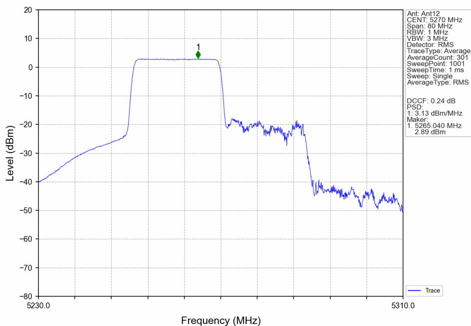
802.11ax(HEW40)_LCH_5270MHz_RU242_Left_Ant12_NTNV
