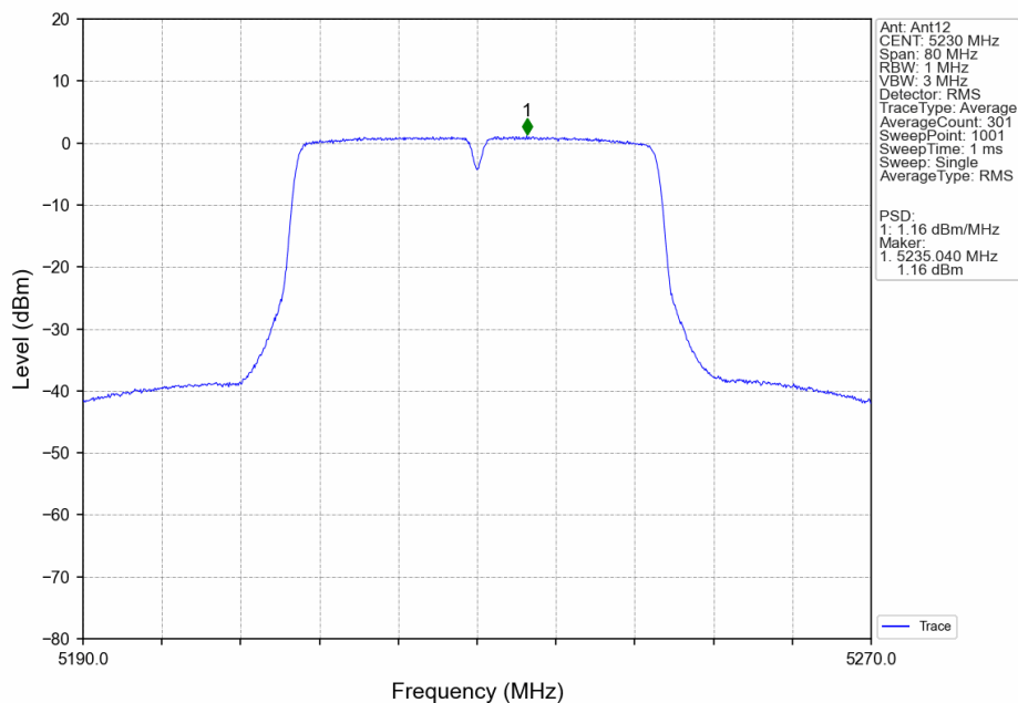
802.11n(HT40)_HCH_5230MHz_Ant12_NTNV
