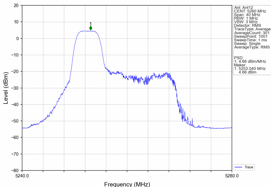
802.11ax(HEW20)_LCH_5260MHz_RU106_Left_Ant12_NTNV
