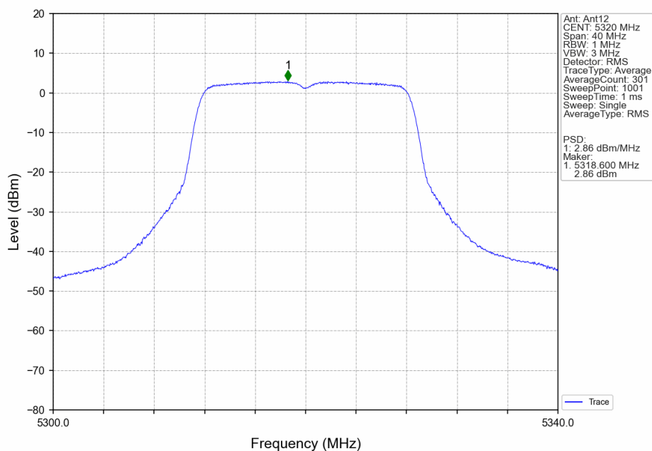
802.11a_HCH_5320MHz_Ant12_NTNV
