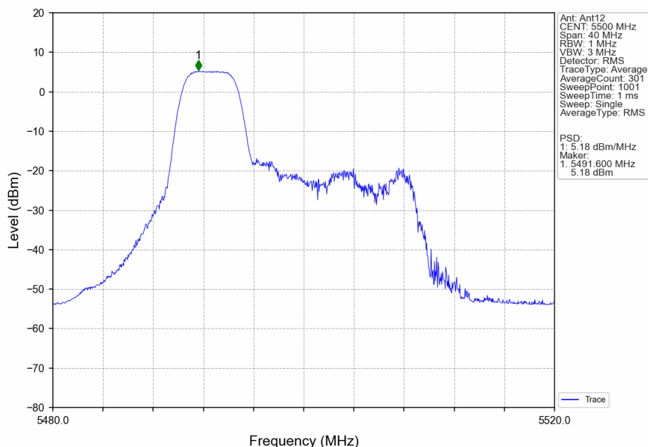
802.11ax(HEW20)_LCH_5500MHz_RU106_Left_Ant12_NTNV
