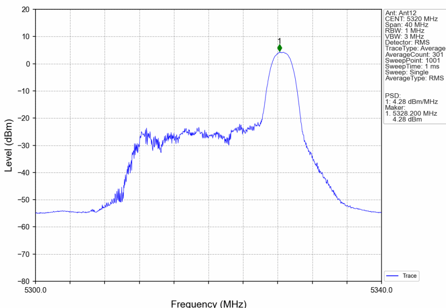
802.11ax(HEW20)_HCH_5320MHz_RU26_Right_Ant12_NTNV
