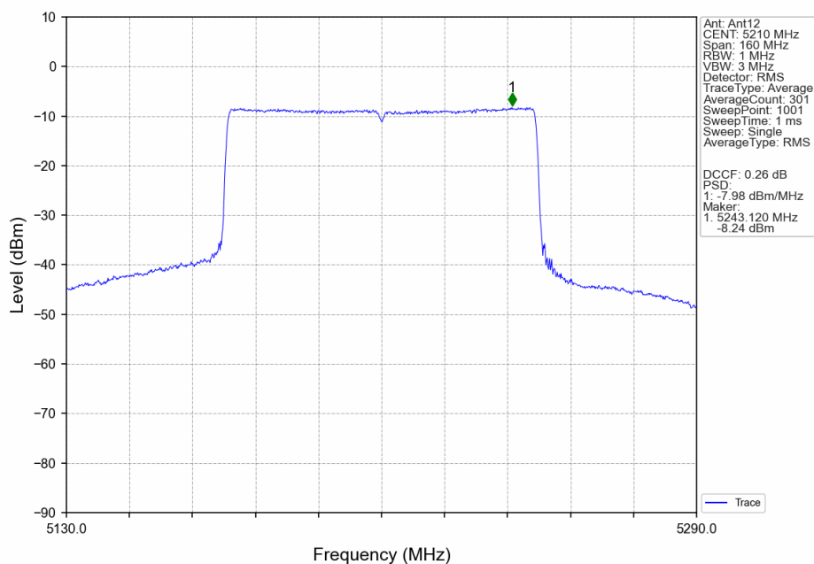
802.11ax(HEW80)_MCH_5210MHz_RU996_Left_Ant12_NTNV
