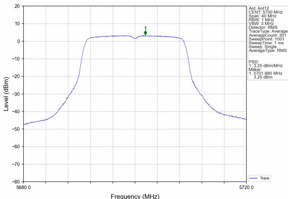
802.11n(HT20)_HCH_5700MHz_Ant12_NTNV
