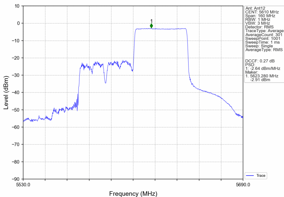
802.11ax(HEW80)_HCH_5610MHz_RU484_Right_Ant12_NTNV
