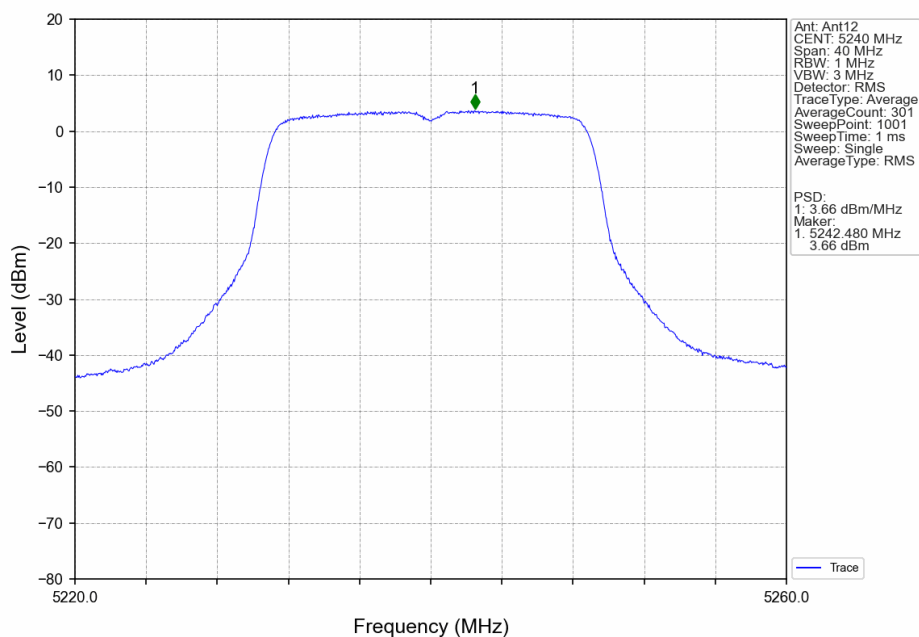
802.11n(HT20)_HCH_5240MHz_Ant12_NTNV
