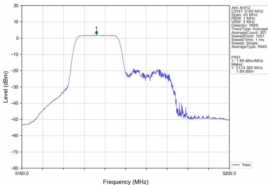
802.11ax(HEW20)_LCH_5180MHz_RU106_Left_Ant12_NTNV
