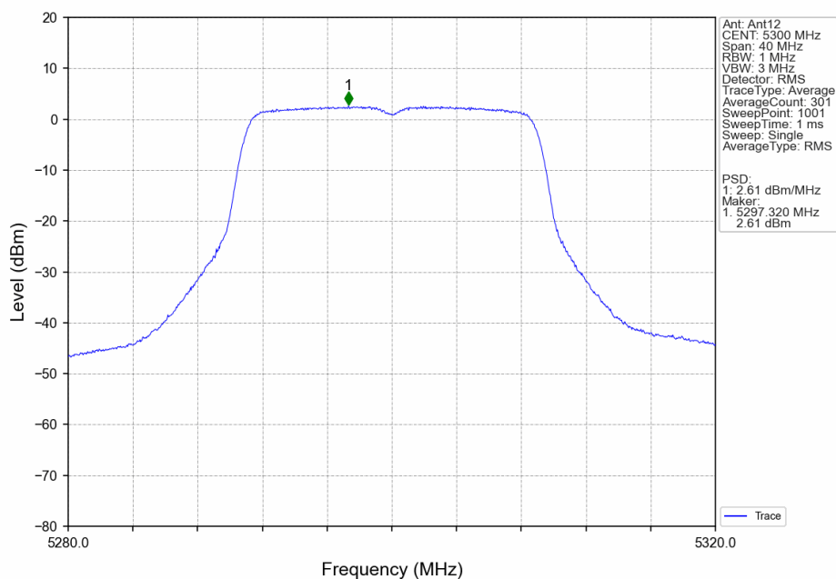
802.11n(HT20)_MCH_5300MHz_Ant12_NTNV
