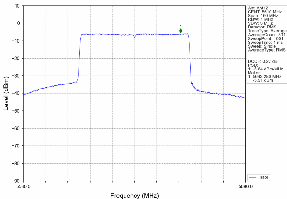
802.11ax(HEW80)_HCH_5610MHz_RU996_Left_Ant12_NTNV
