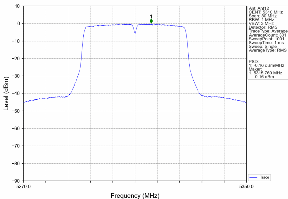
802.11n(HT40)_HCH_5310MHz_Ant12_NTNV
