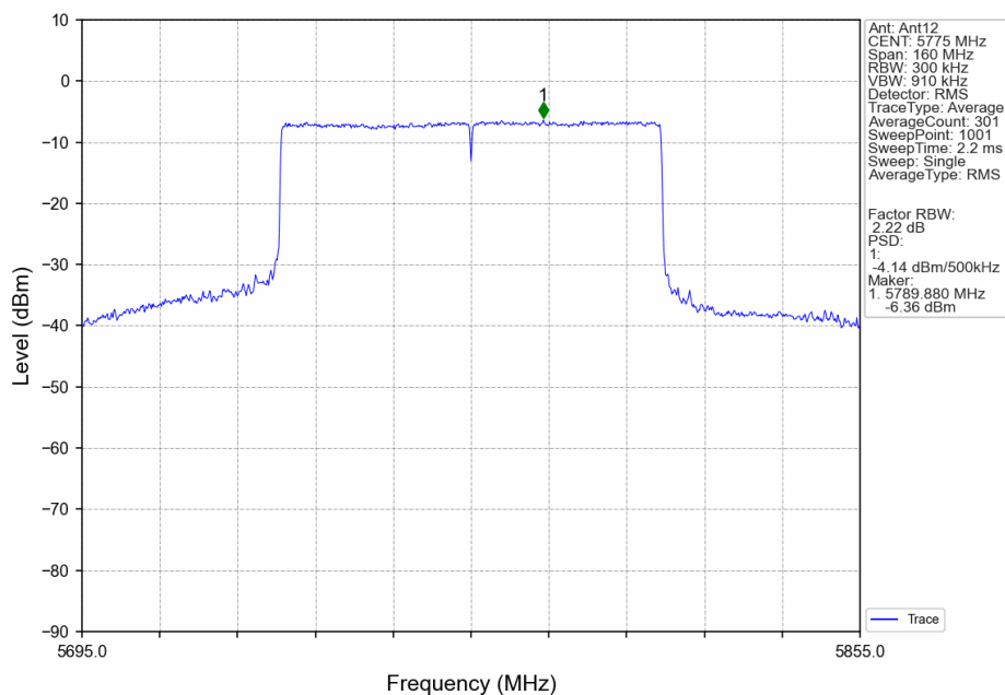
802.11ax(HEW80)_MCH_5775MHz_RU996_Left_Ant12_NTNV
