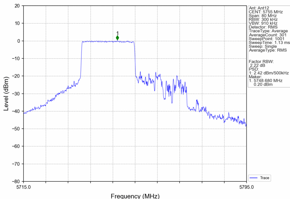
802.11ax(HEW40)_LCH_5755MHz_RU484_Left_Ant12_NTNV
