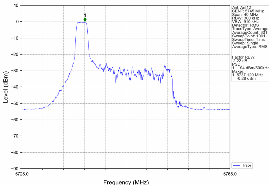
802.11ax(HEW20)_LCH_5745MHz_RU52_Left_Ant12_NTNV
