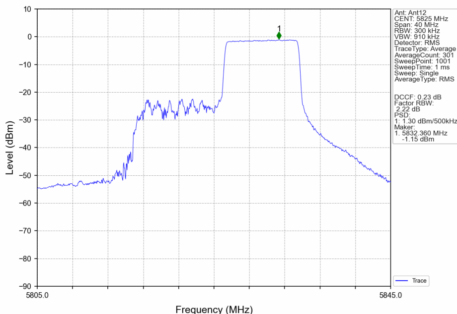
802.11ax(HEW20)_HCH_5825MHz_RU242_Left_Ant12_NTNV
