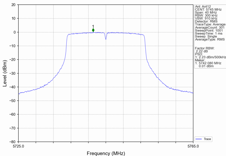
802.11n(HT20)_LCH_5745MHz_Ant12_NTNV
