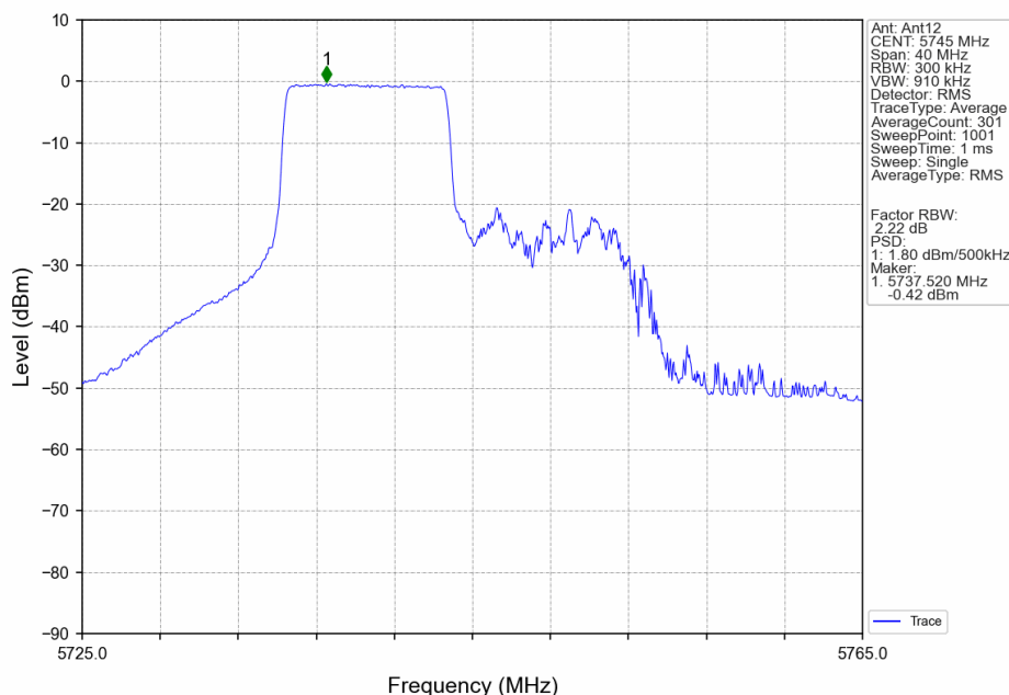
802.11ax(HEW20)_LCH_5745MHz_RU242_Left_Ant12_NTNV
