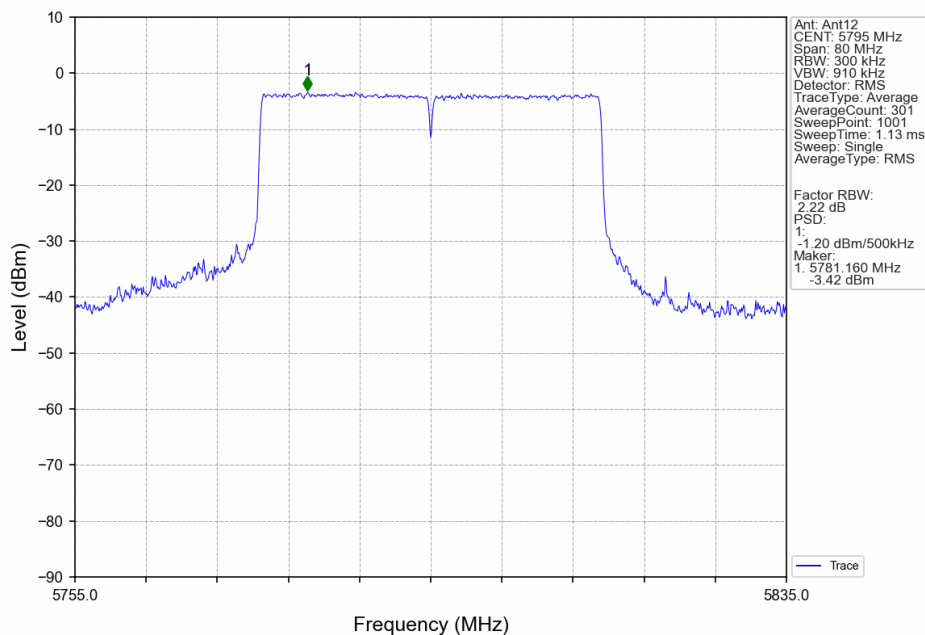
802.11ax(HEW40)_HCH_5795MHz_RU484_Left_Ant12_NTNV
