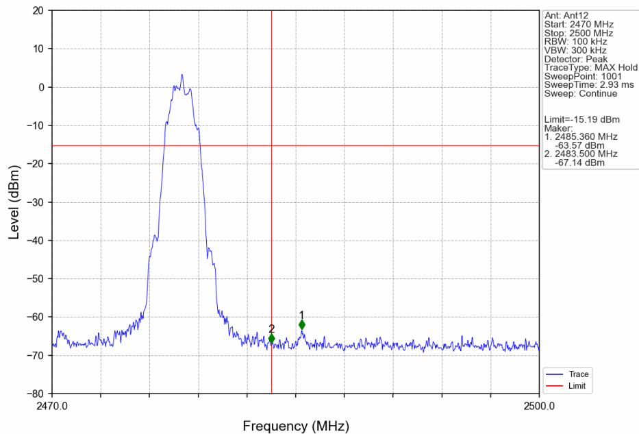
2M_HCH_2478MHz_Ant12_NTNV
