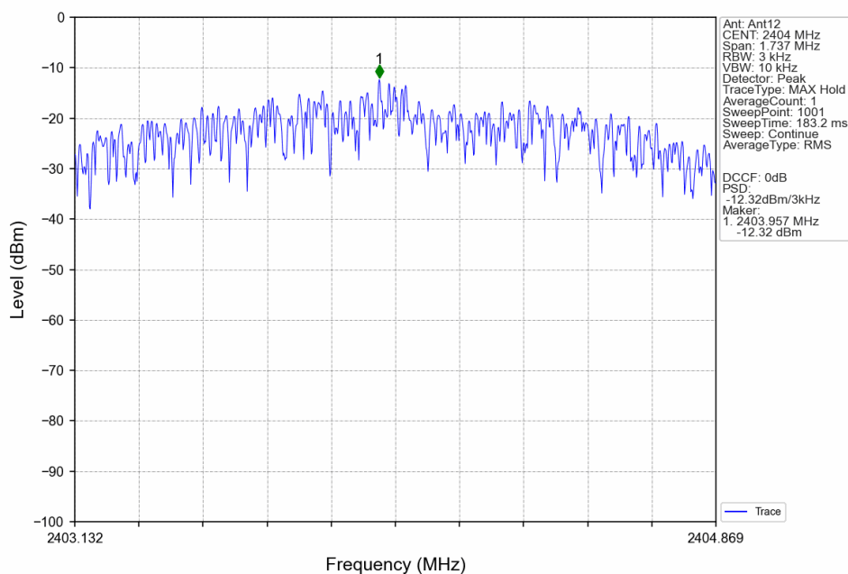
2M_LCH_2404MHz_Ant12_NTNV
