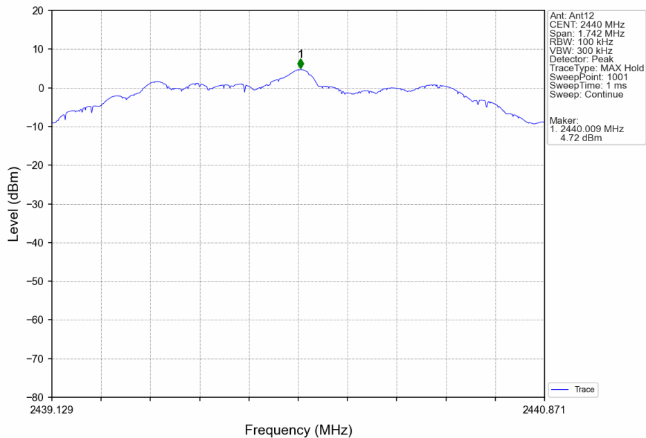
2M_MCH_2440MHz_Ant12_NTNV
