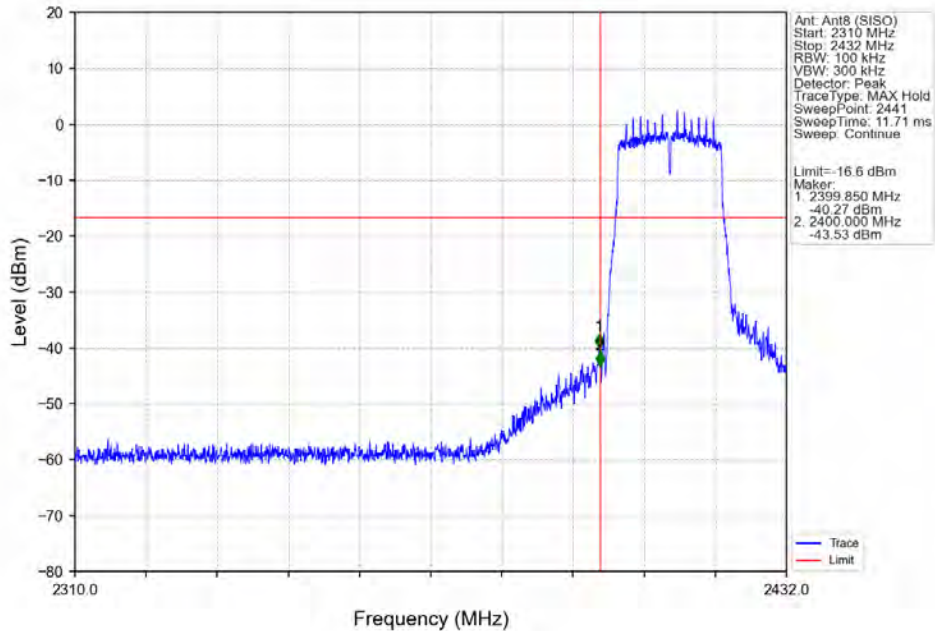
802.11n(HT20)_LCH_2412MHz_Ant8 (SISO)_NTNV
