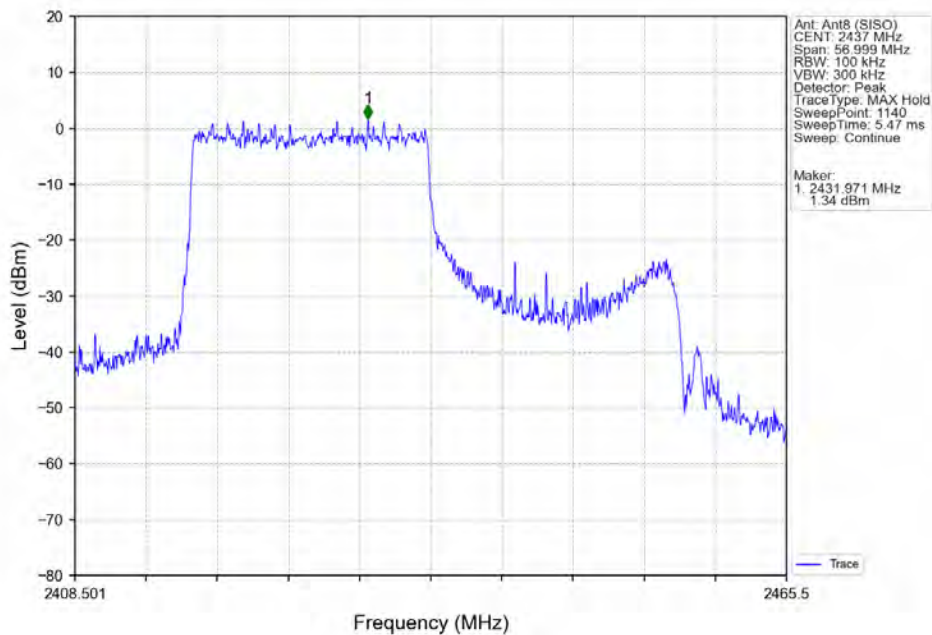
802.11ax(HEW40)_MCH_2437MHz_RU242_Left_Ant8 (SISO)_NTNV
