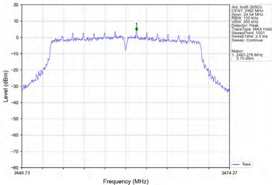
802.11VHT(VHT20)_HCH_2462MHz_Ant8 (SISO)_NTNV
