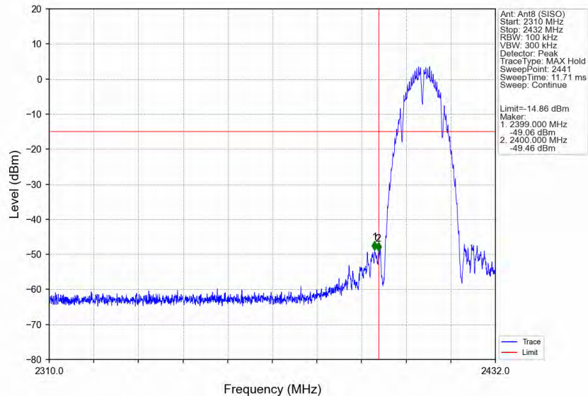
802.11b_LCH_2412MHz_Ant8 (SISO)_NTNV
