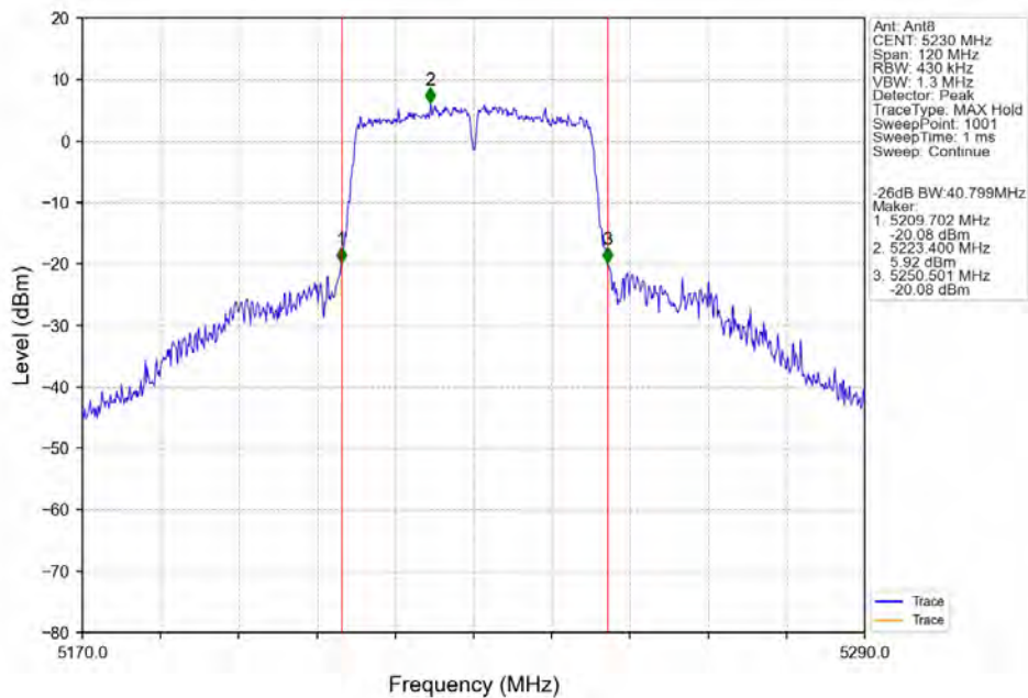
802.11ac(VHT40)_HCH_5230MHz_Ant8_NTNV
