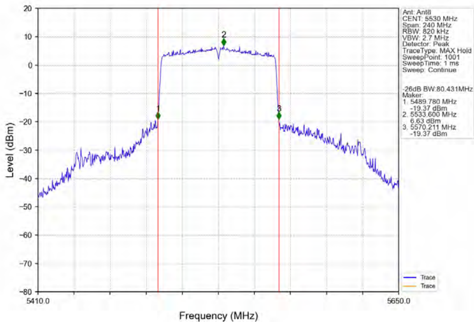
802.11ac(VHT80)_LCH_5530MHz_Ant8_NTNV
