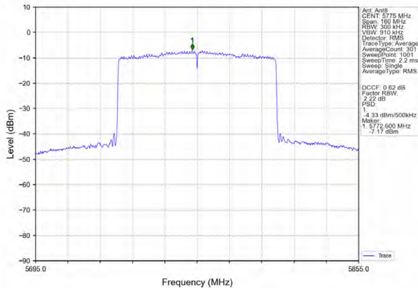
802.11ax(HEW80)_MCH_5775MHz_RU996_Left_Ant8_NTNV
