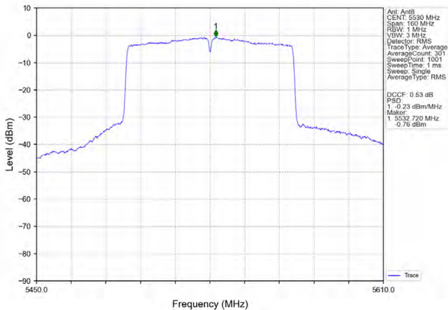
802.11ac(VHT80)_LCH_5530MHz_Ant8_NTNV
