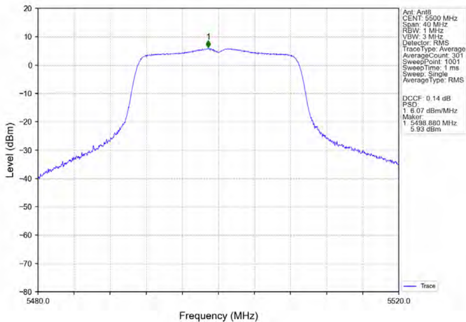
802.11n(HT20)_LCH_5500MHz_Ant8_NTNV
