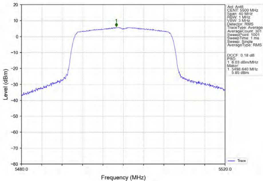
802.11ax(HEW20)_LCH_5500MHz_RU242_Left_Ant8_NTNV
