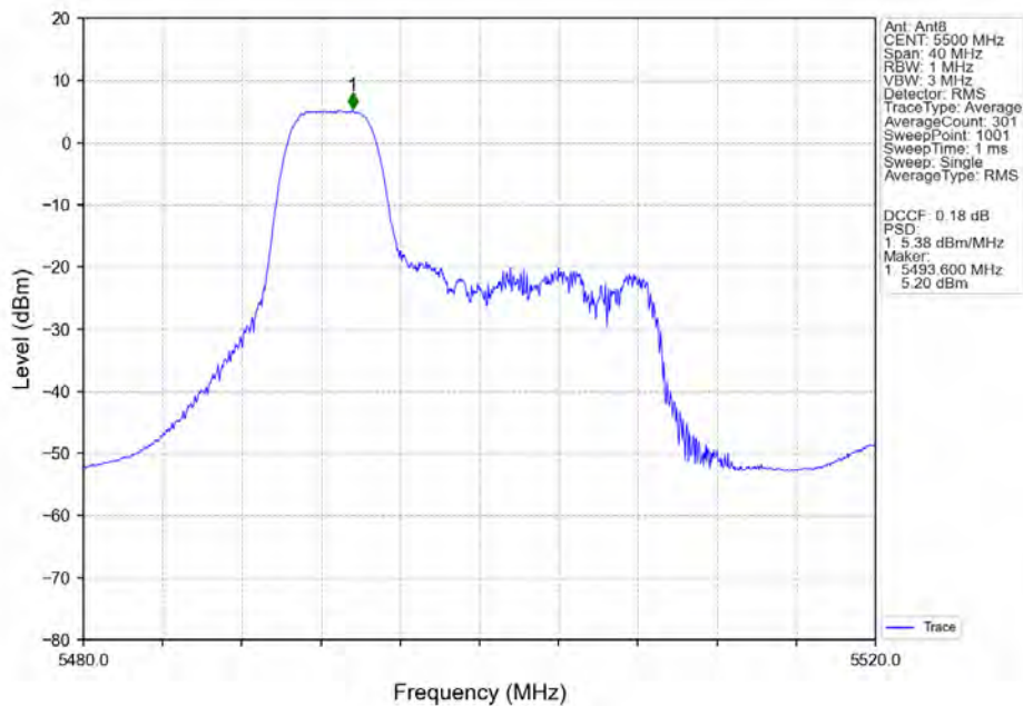
802.11ax(HEW20)_LCH_5500MHz_RU52_Left_Ant8_NTNV
