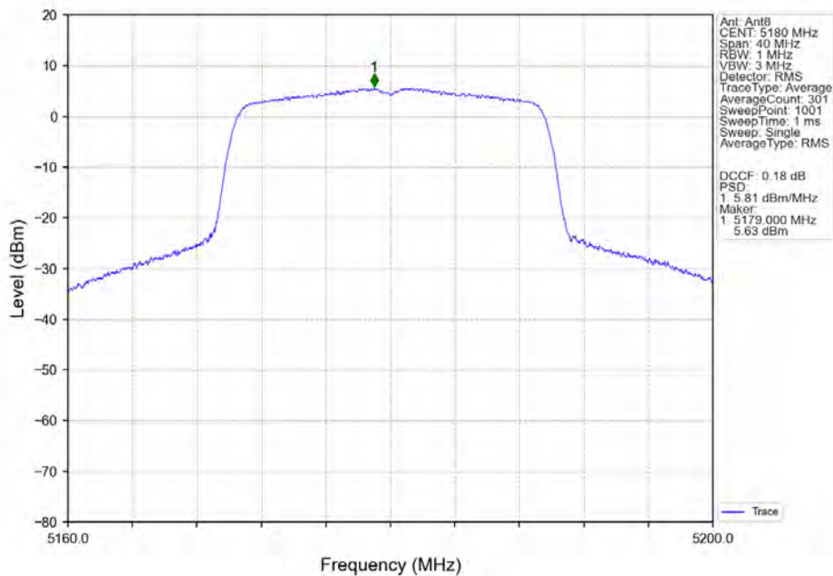
802.11ax(HEW20)_LCH_5180MHz_RU242_Left_Ant8_NTNV
