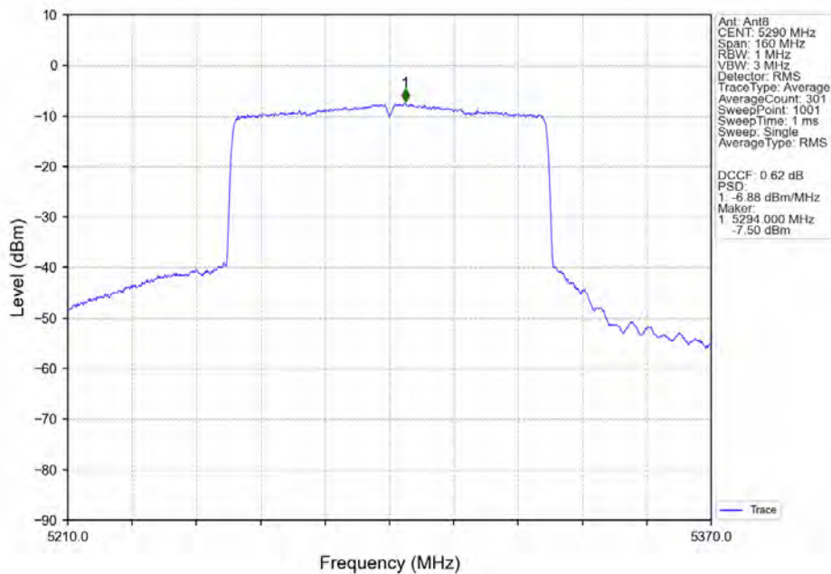
802.11ax(HEW80)_MCH_5290MHz_RU996_Left_Ant8_NTNV
