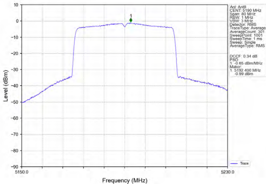
802.11ax(HEW40)_LCH_5190MHz_RU484_Left_Ant8_NTNV
