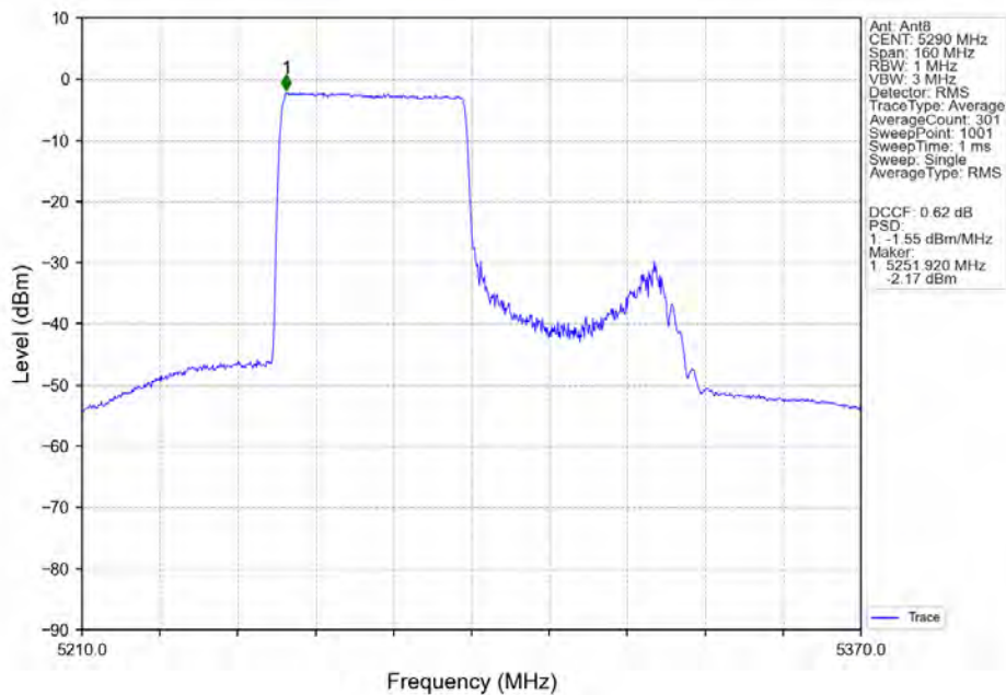
802.11ax(HEW80)_MCH_5290MHz_RU484_Left_Ant8_NTNV
