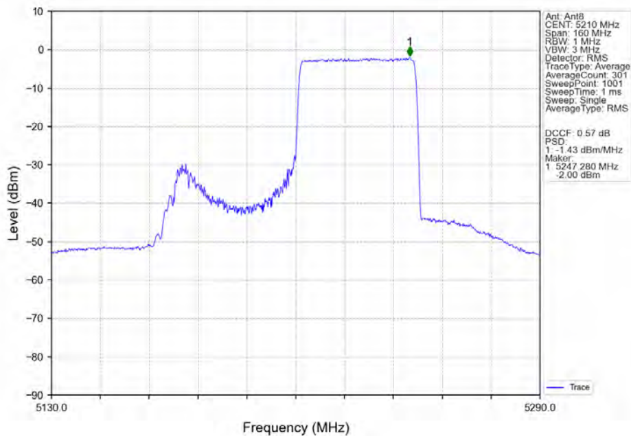
802.11ax(HEW80)_MCH_5210MHz_RU484_Right_Ant8_NTNV
