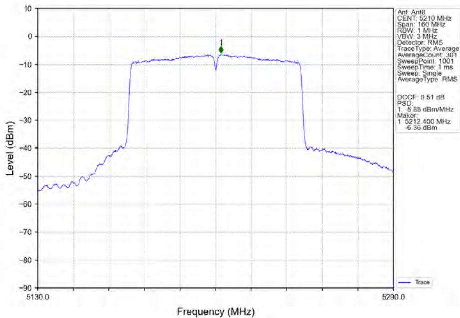
802.11ac(VHT80)_MCH_5210MHz_Ant8_NTNV
