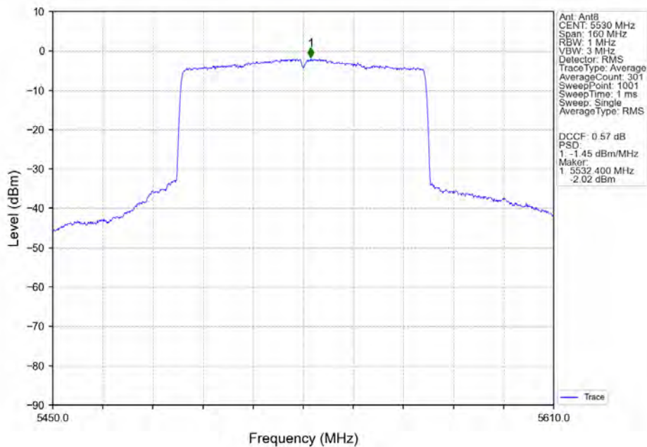
802.11ax(HEW80)_LCH_5530MHz_RU996_Left_Ant8_NTNV
