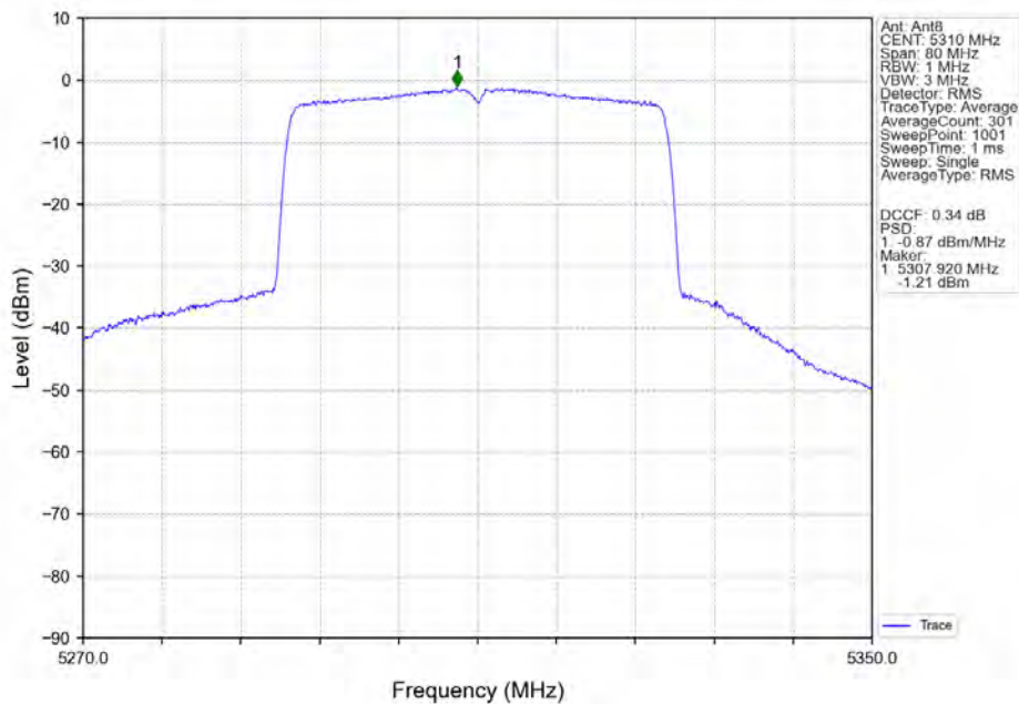
802.11ax(HEW40)_HCH_5310MHz_RU484_Left_Ant8_NTNV
