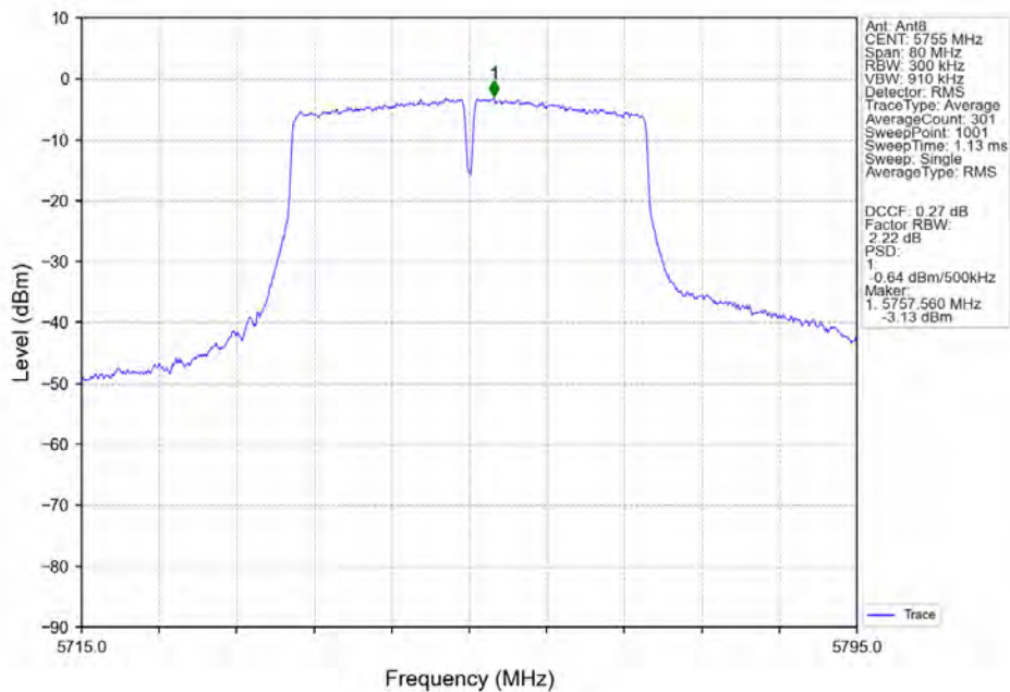
802.11ac(VHT40)_LCH_5755MHz_Ant8_NTNV
