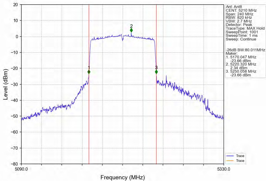
802.11ac(VHT80)_MCH_5210MHz_Ant8_NTNV
