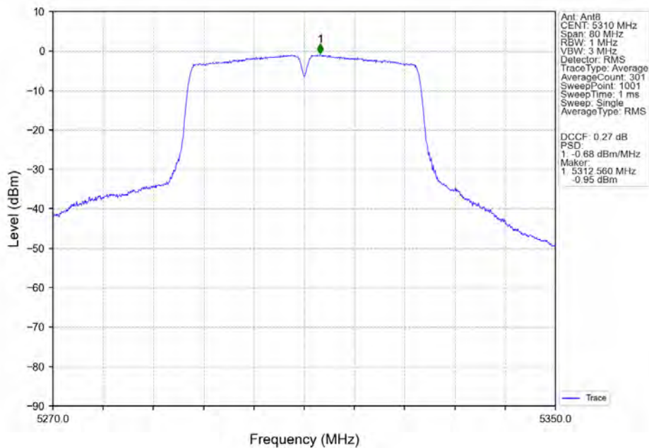
802.11n(HT40)_HCH_5310MHz_Ant8_NTNV
