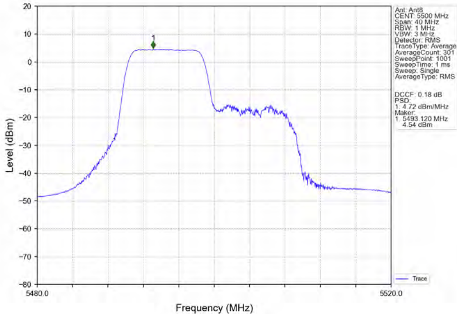
802.11ax(HEW20)_LCH_5500MHz_RU242_Left_Ant8_NTNV
