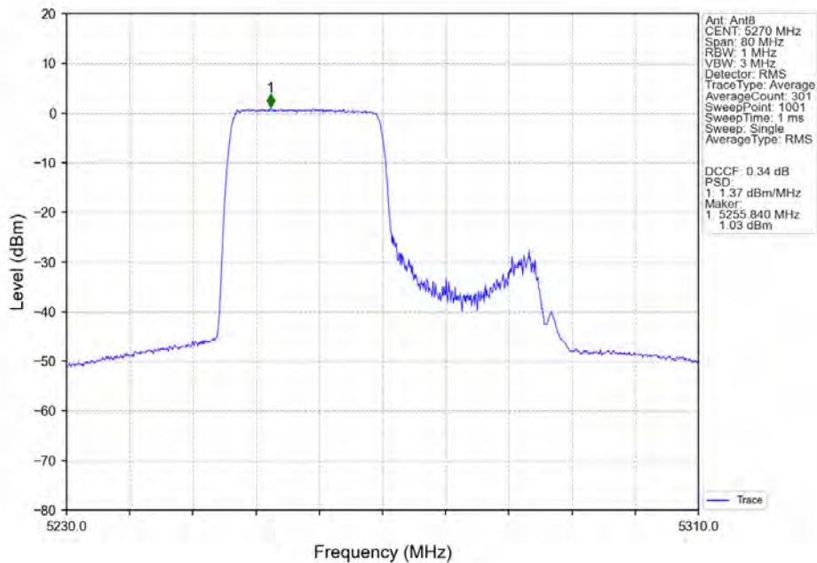
802.11ax(HEW40)_LCH_5270MHz_RU484_Left_Ant8_NTNV
