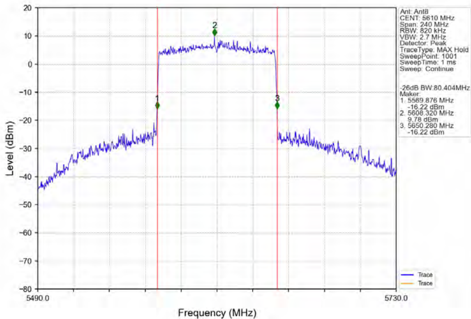
802.11ax(HEW80)_HCH_5610MHz_RU996_Left_Ant8_NTNV
