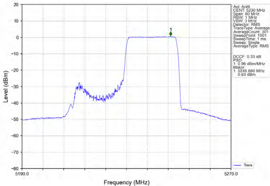
802.11ax(HEW40)_HCH_5230MHz_RU484_Left_Ant8_NTNV
