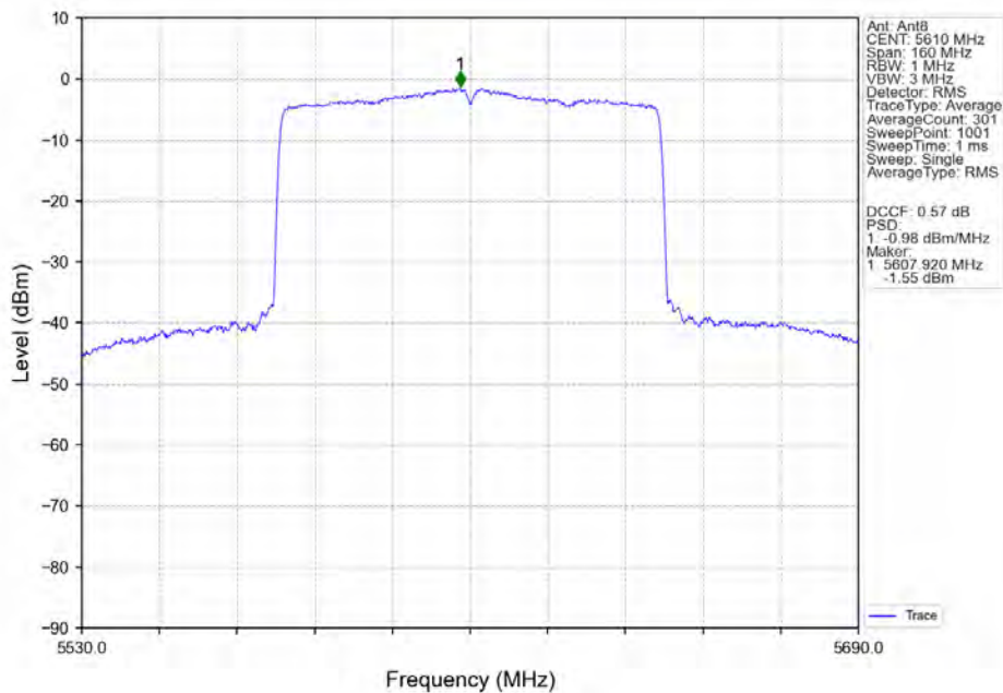
802.11ax(HEW80)_HCH_5610MHz_RU996_Left_Ant8_NTNV
