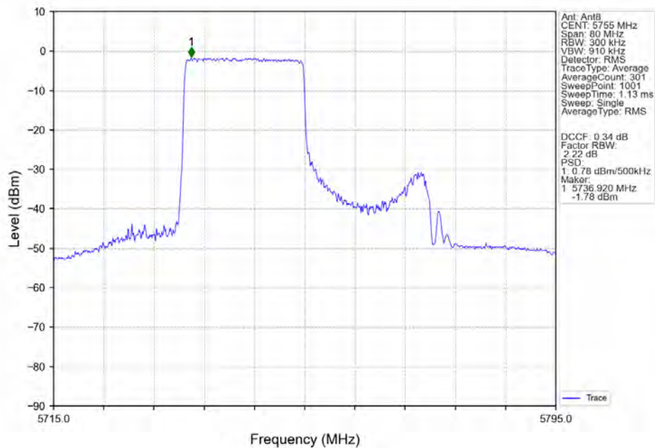
802.11ax(HEW40)_LCH_5755MHz_RU242_Left_Ant8_NTNV
