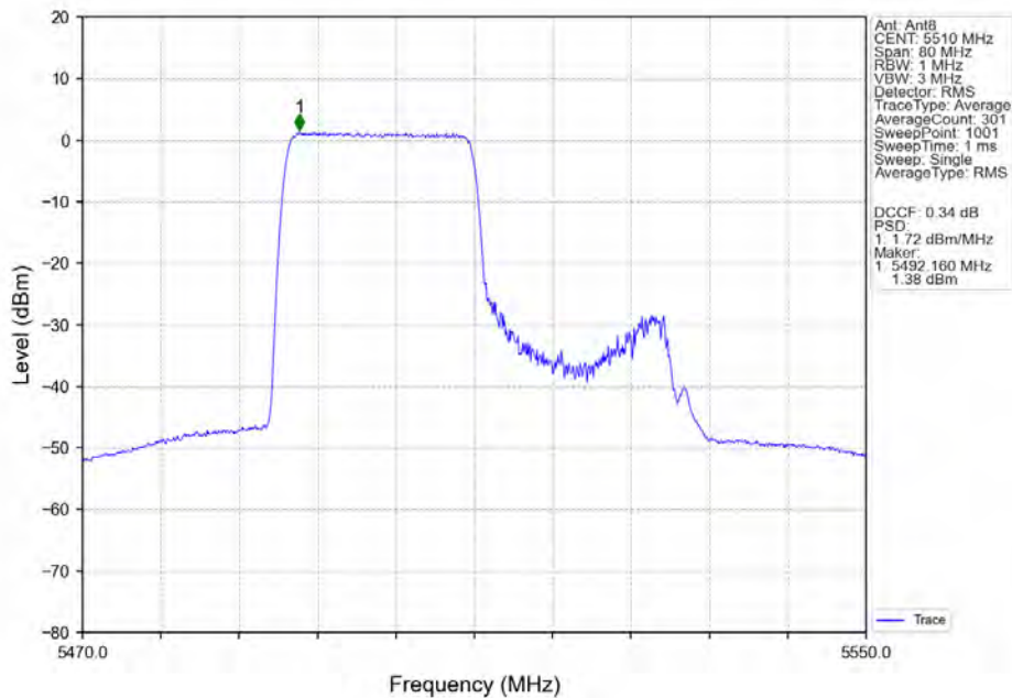
802.11ax(HEW40)_LCH_5510MHz_RU484_Left_Ant8_NTNV
