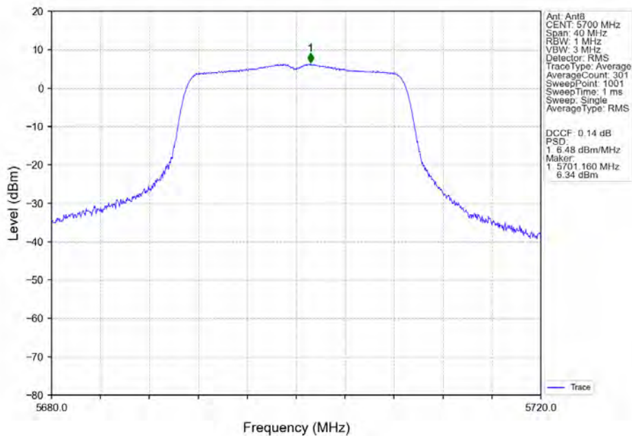
802.11ac(VHT20)_HCH_5700MHz_Ant8_NTNV
