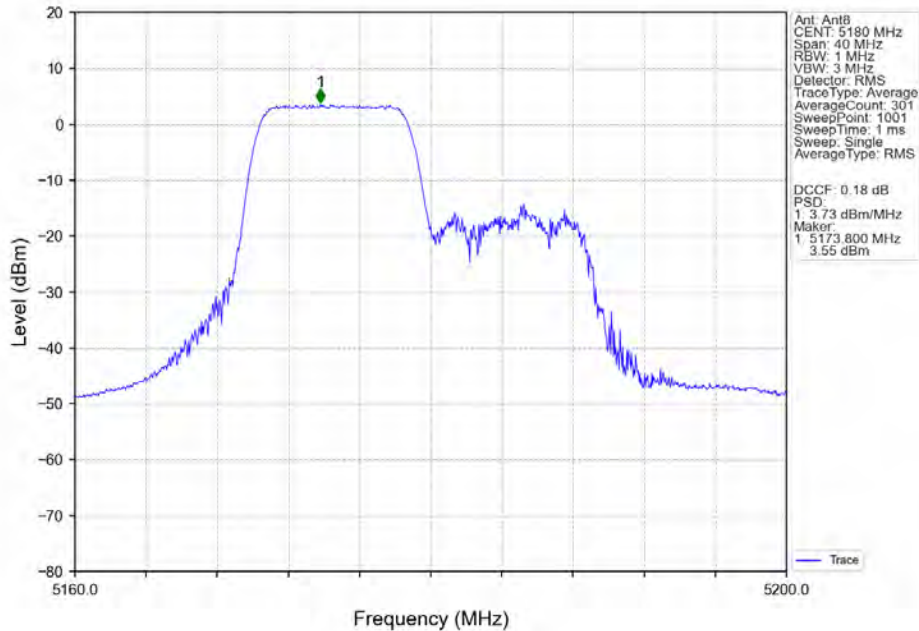
802.11ax(HEW20)_LCH_5180MHz_RU242_Left_Ant8_NTNV
