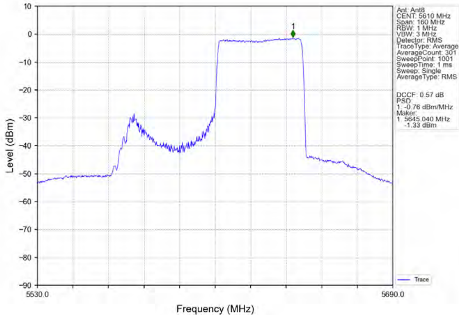
802.11ax(HEW80)_HCH_5610MHz_RU996_Left_Ant8_NTNV
