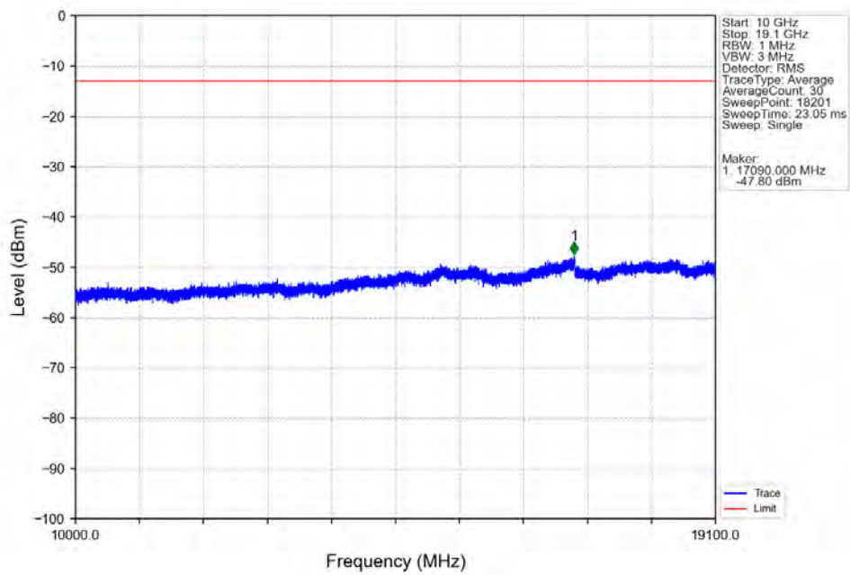
Band2 10MHz 64QAM MCH 1880MHz RB 1 0 NTNV
