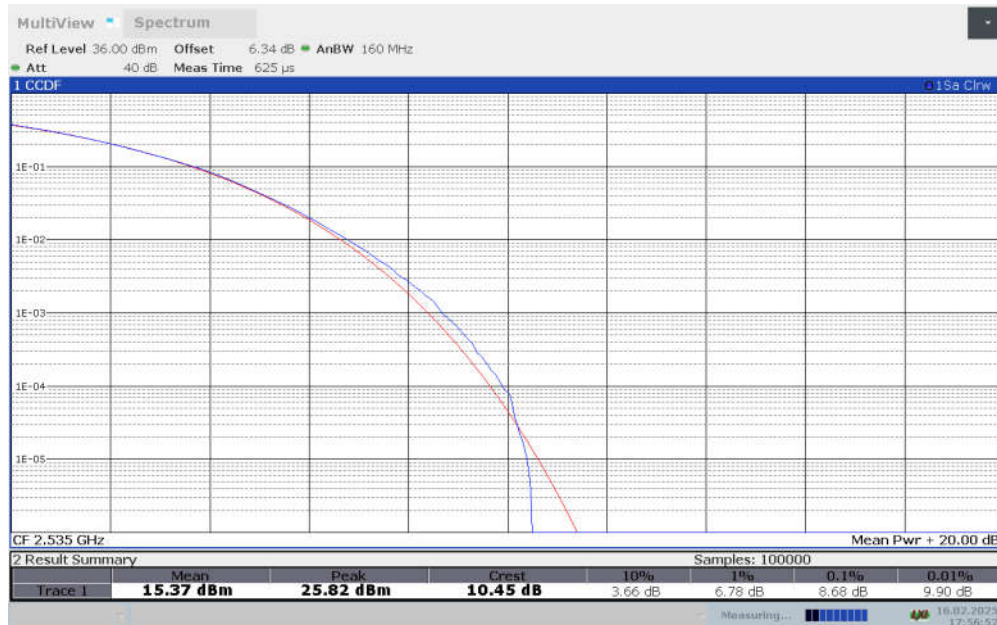
n7, CP-QPSK (PAPR)
