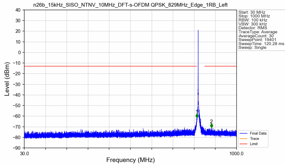
n26b_15kHz_SISO_NTNV_10MHz_DFT-s-OFDM QPSK_829MHz_Edge_1RB_Left_Ant0
