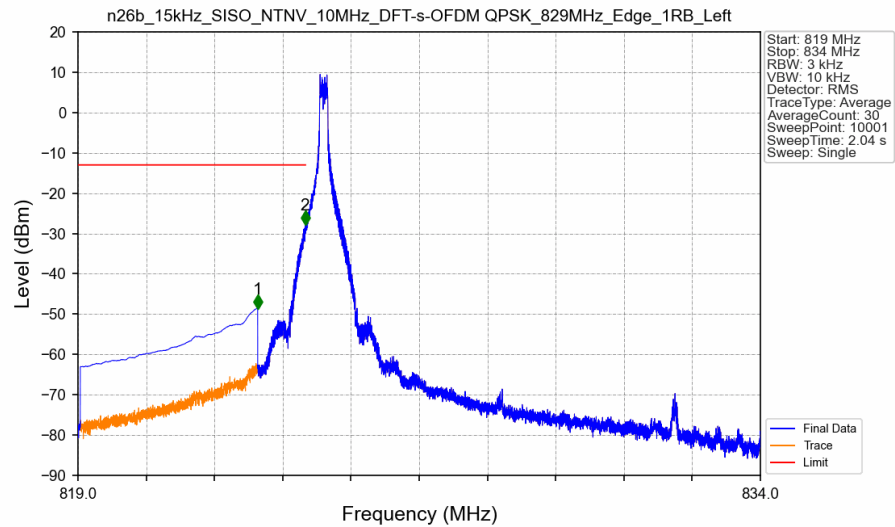
n26b_15kHz_SISO_NTNV_10MHz_DFT-s-OFDM QPSK_829MHz_Edge_1RB_Left_Ant0
