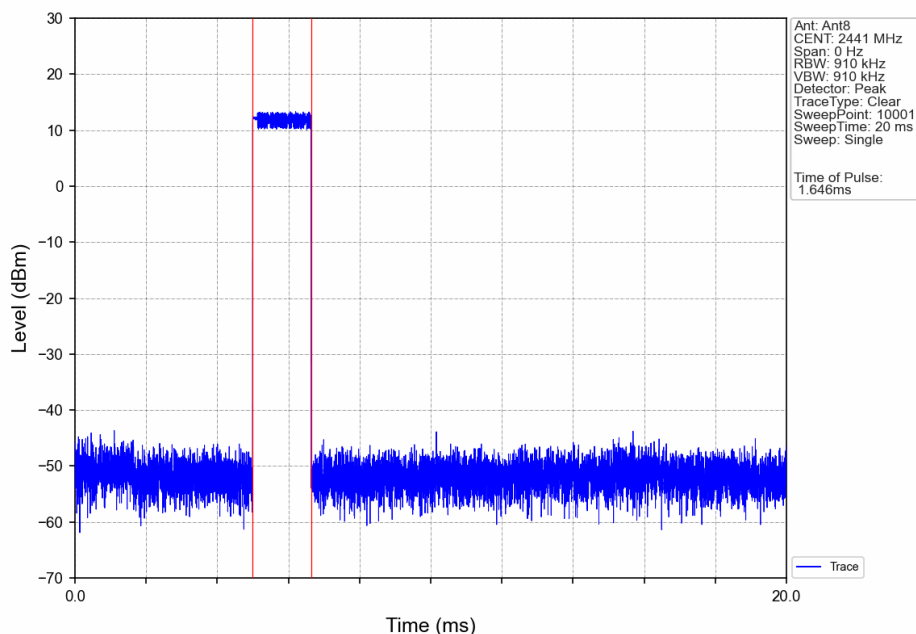
Pi/4DQPSK_2DH3_HOPP_Ant8_NTNV
