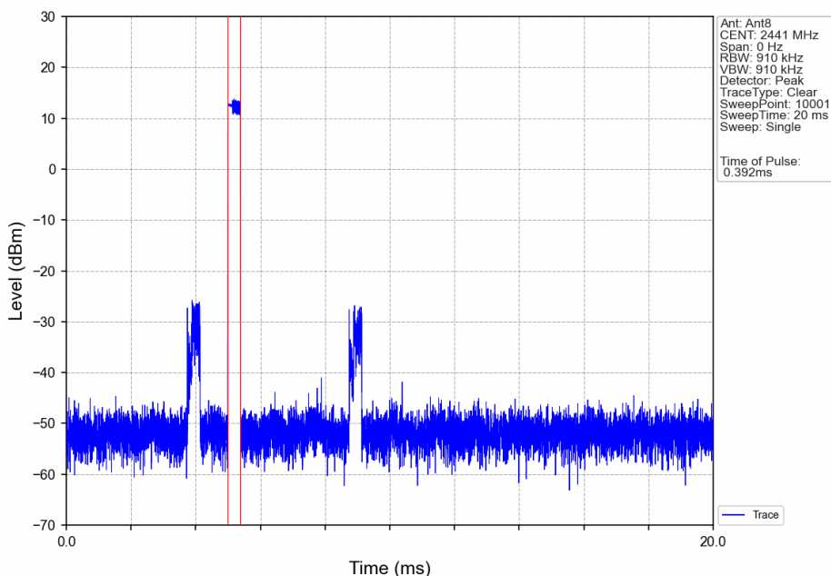
Pi/4DQPSK_2DH1_HOPP_Ant8_NTNV
