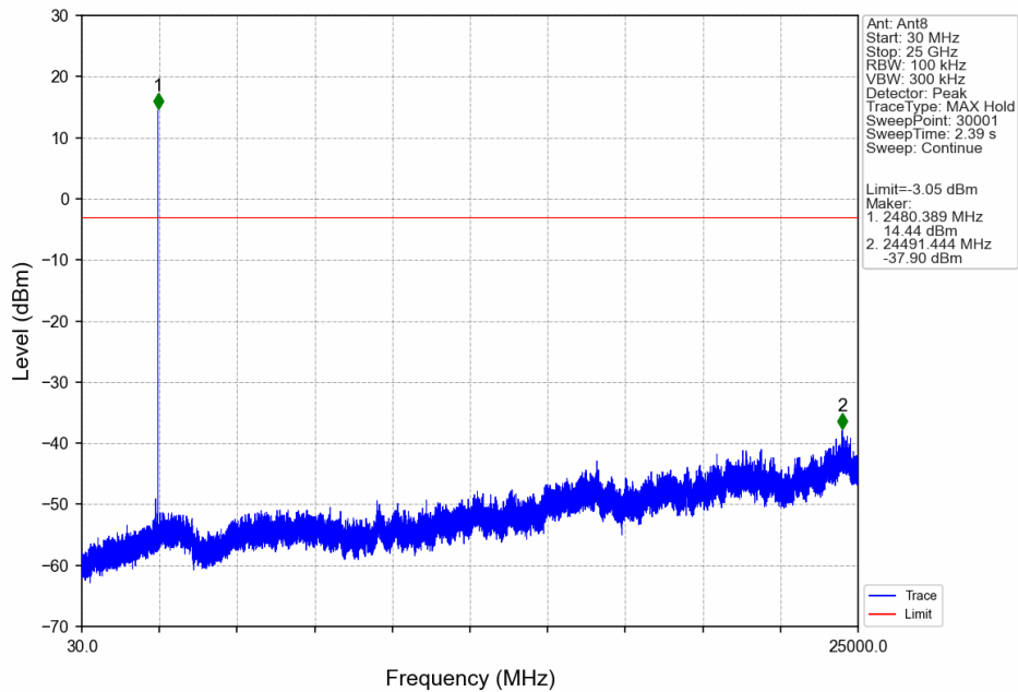
GFSK_DH5_HOPP_Ant8_NTNV
