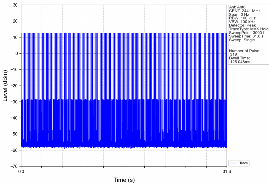
Pi/4DQPSK_2DH1_HOPP_Ant8_NTNV
