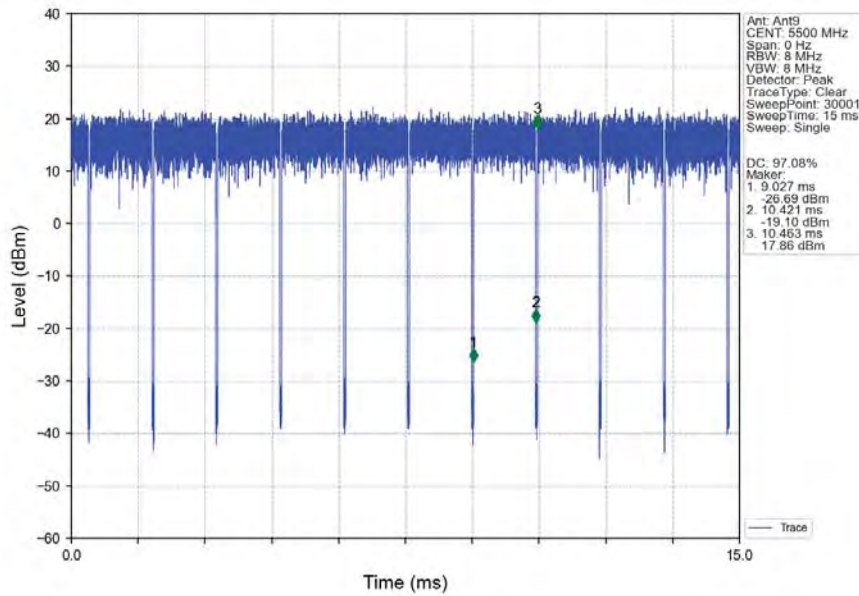
802.11a_LCH_5500MHz_Ant9_NTNV
