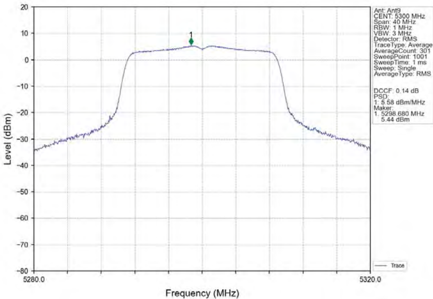
802.11n(HT20)_MCH_5300MHz_Ant9_NTNV
