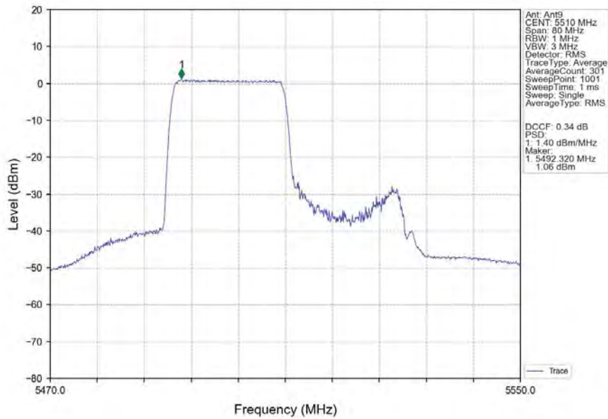
802.11ax(HEW40)_LCH_5510MHz_RU242_Left_Ant9_NTNV
