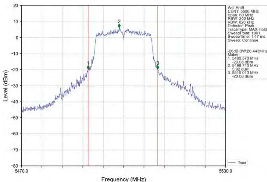
802.11a_LCH_5500MHz_Ant9_NTNV
