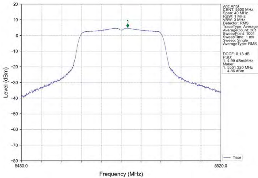
802.11a_LCH_5500MHz_Ant9_NTNV
