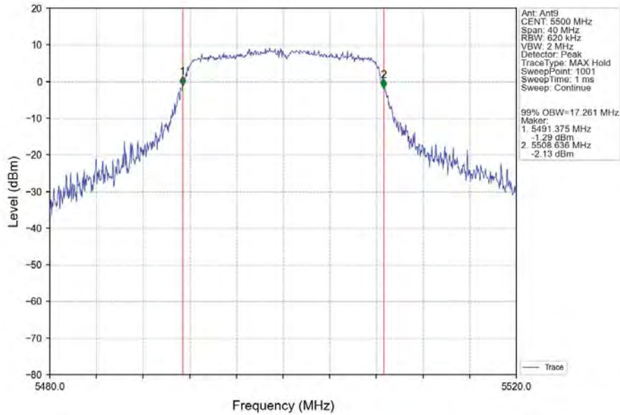
802.11a_LCH_5500MHz_Ant9_NTNV
