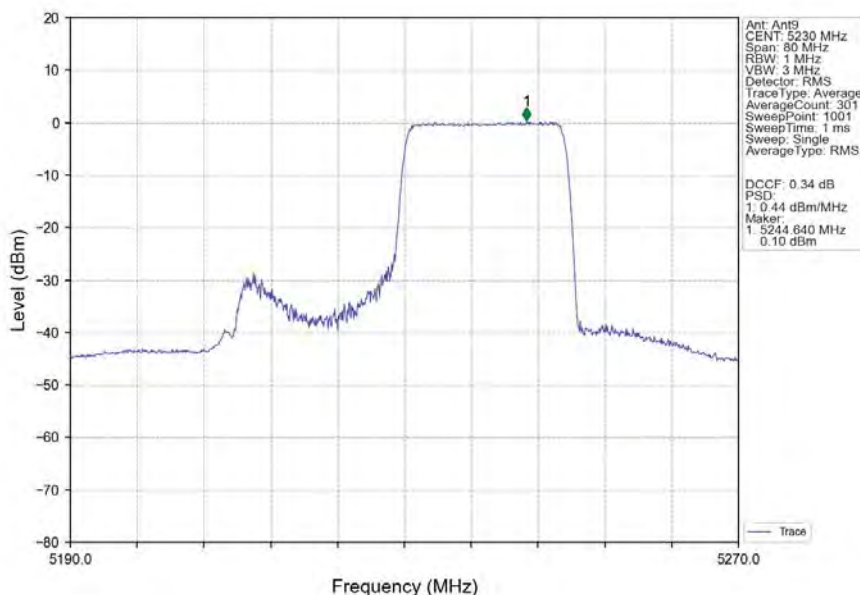
802.11ax(HEW40)_HCH_5230MHz_RU242_Right_Ant9_NTNV
