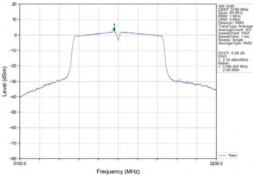
802.11n(HT40)_LCH_5190MHz_Ant9_NTNV
