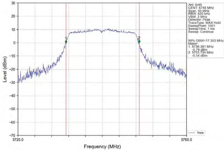
802.11a_LCH_5745MHz_Ant9_NTNV
