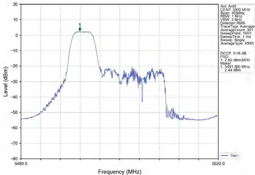
802.11ax(HEW20)_LCH_5500MHz_RU52_Left_Ant9_NTNV
