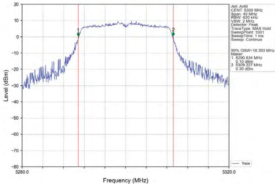
802.11n(HT20)_MCH_5300MHz_Ant9_NTNV
