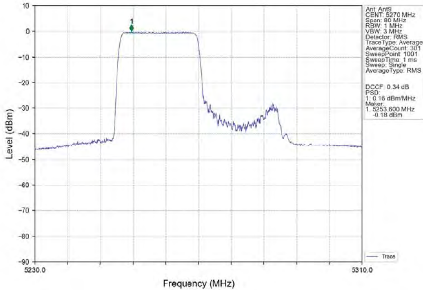
802.11ax(HEW40)_LCH_5270MHz_RU242_Left_Ant9_NTNV
