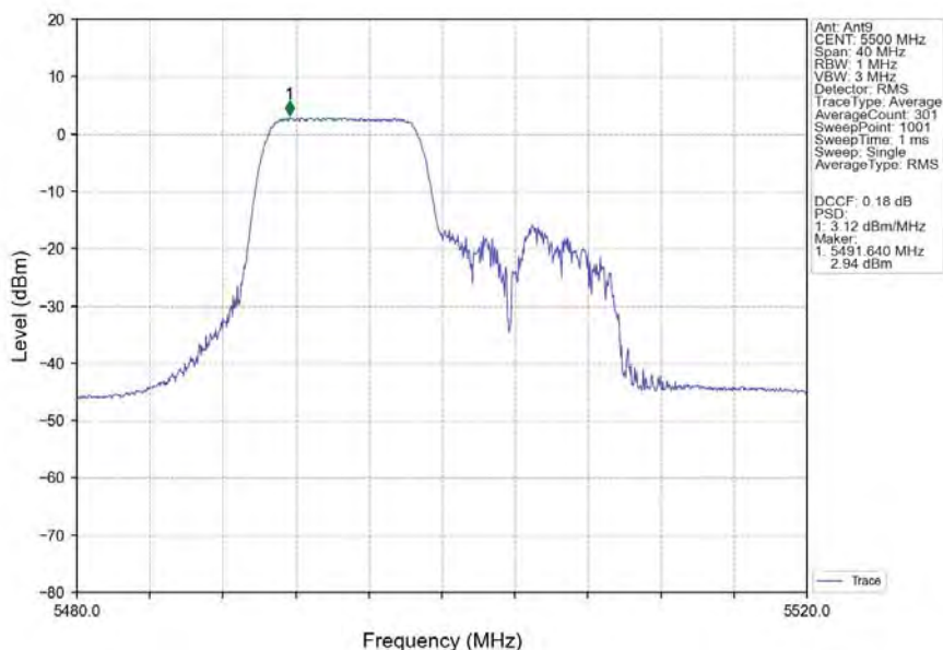
802.11ax(HEW20)_LCH_5500MHz_RU106_Left_Ant9_NTNV
