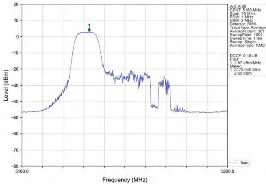
802.11ax(HEW20)_LCH_5180MHz_RU52_Left_Ant9_NTNV
