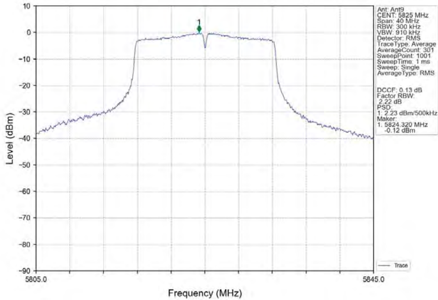
802.11a_HCH_5825MHz_Ant9_NTNV
