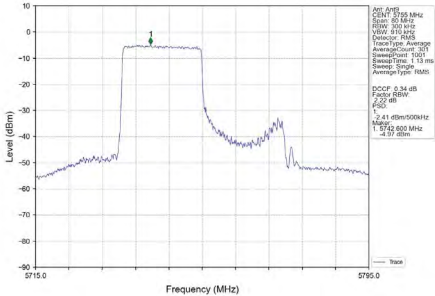
802.11ax(HEW40)_LCH_5755MHz_RU242_Left_Ant9_NTNV
