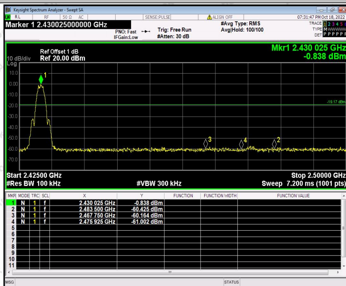
2.4g_Ant1_Low_2430
