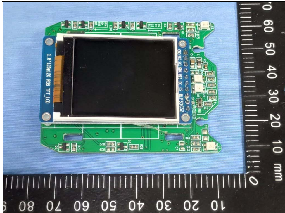
PCB-3
