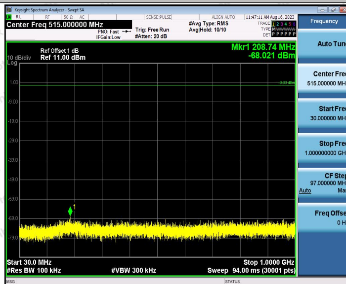
2.4G_Ant1_2442_30~1000
