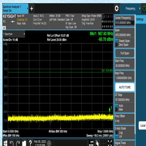
2DH5-Ant1-2402-30~1000-6.20
