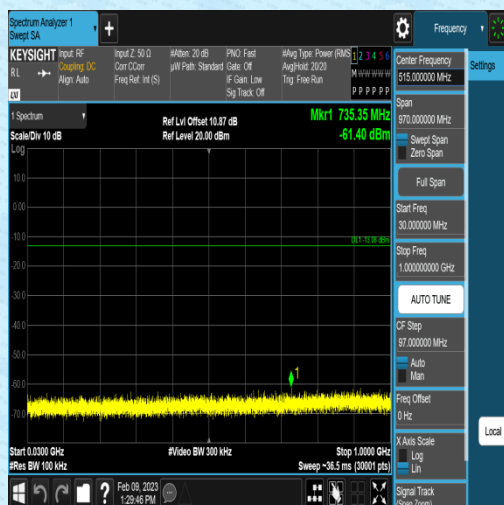
DH5-Ant1-2402-30~1000-6.92
