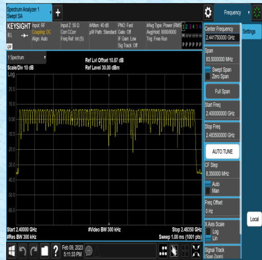
DH5-Ant1-Hop
